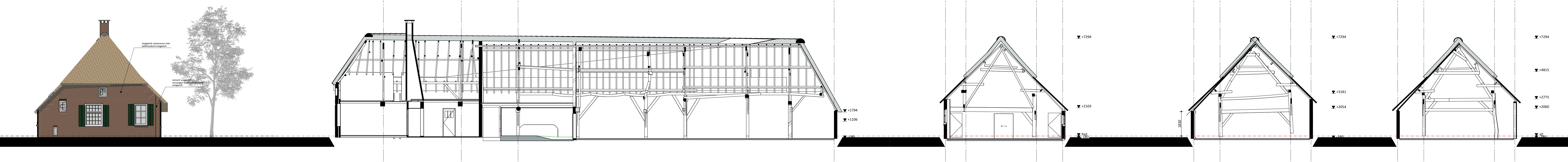
doorsnede A-A
