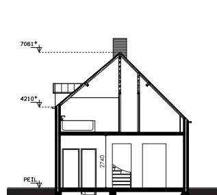
DOORSNEDE D-D
