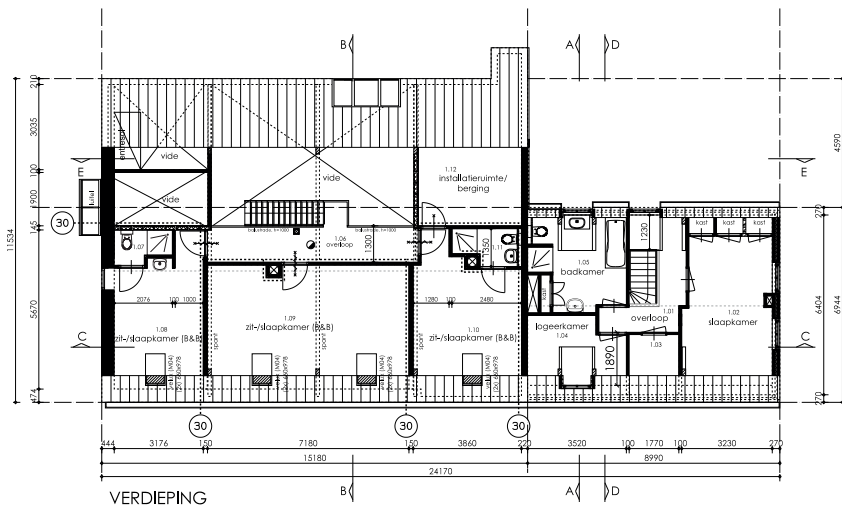
VERDIEPING
