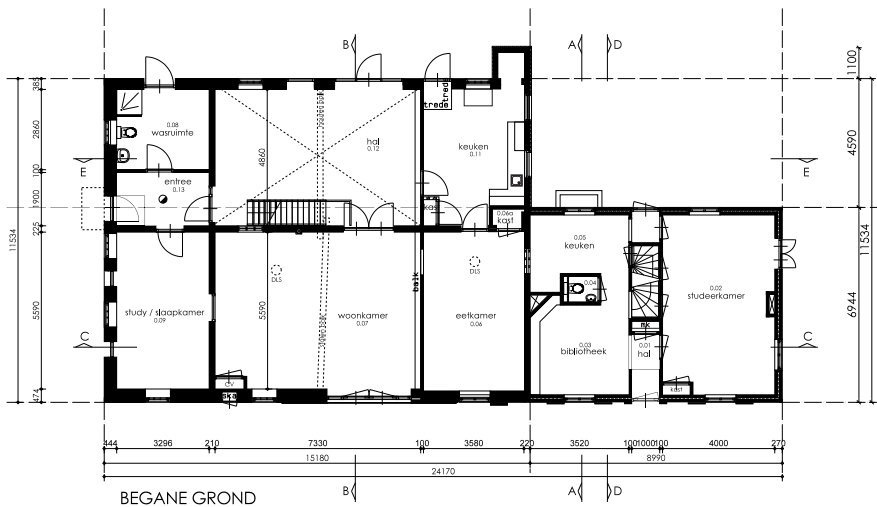
BEGANE GROND
