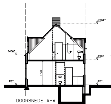
DOORSNEDE A-A
