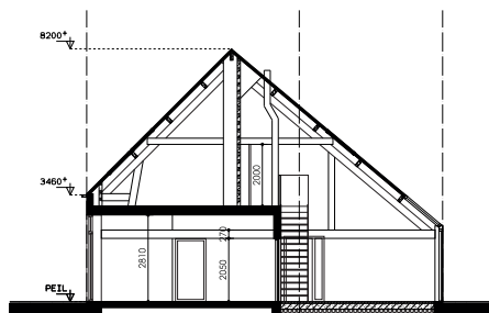
DOORSNEDE B-B
