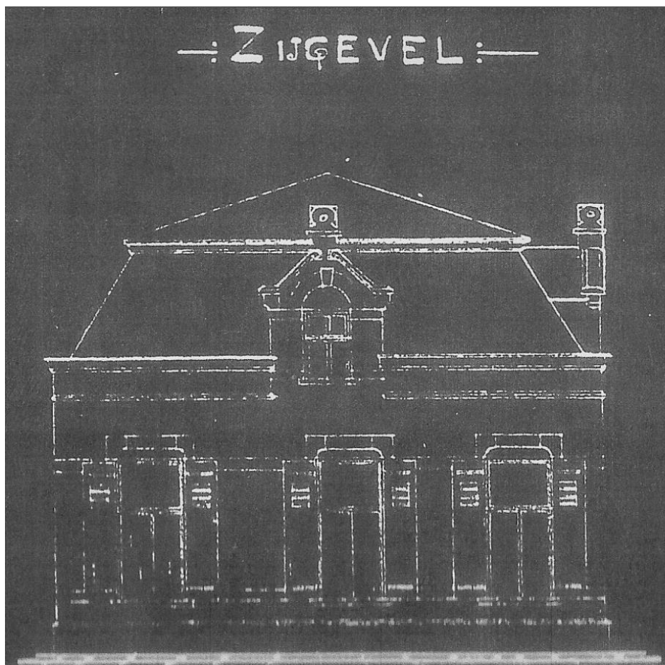
Blauwdruk uit 1905 van de linker zijgevel van de woning. Kopie Coll. Fam. Van Roosmalen.
