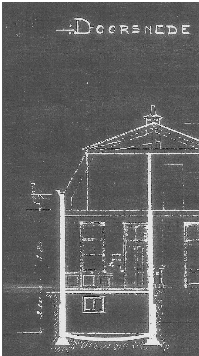
Blauwdruk uit 1905 van de keuken met onderkeldering van de woning. Kopie Coll. Fam. Van Roosmalen.
