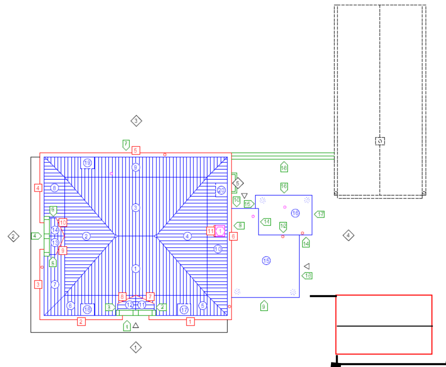
Dakplattegronden van het huis met aanbouwen met in groen de erfmuur en gestippeld het bakhuis/annex schuur. In rood omlijnd de garage uit 1962. Bron: Monumentenwacht Brabant, aanvulling FH MAB.
