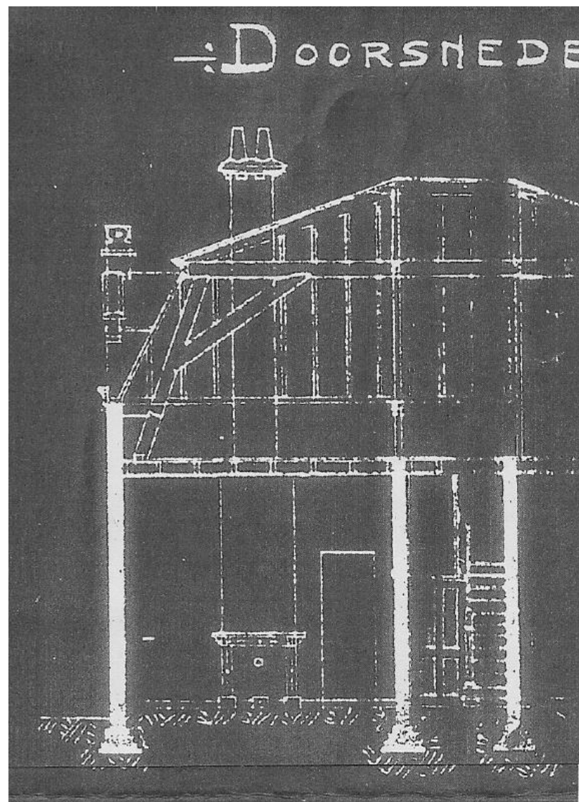
Blauwdruk uit 1905 van de doorsnede over de linker voorkamer en gang van de woning. Kopie Coll. Fam. Van Roosmalen.
