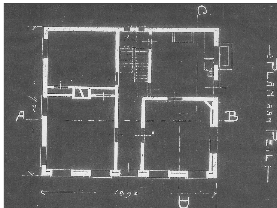
Blauwdruk uit 1905 van de plattegrond begane grond van de woning. De voorgevel is beneden. Let op de getekende spouwmuur bij de voorgevel en een deel van de rechter zijgevel! Kopie Coll. Fam. Van Roosmalen.
