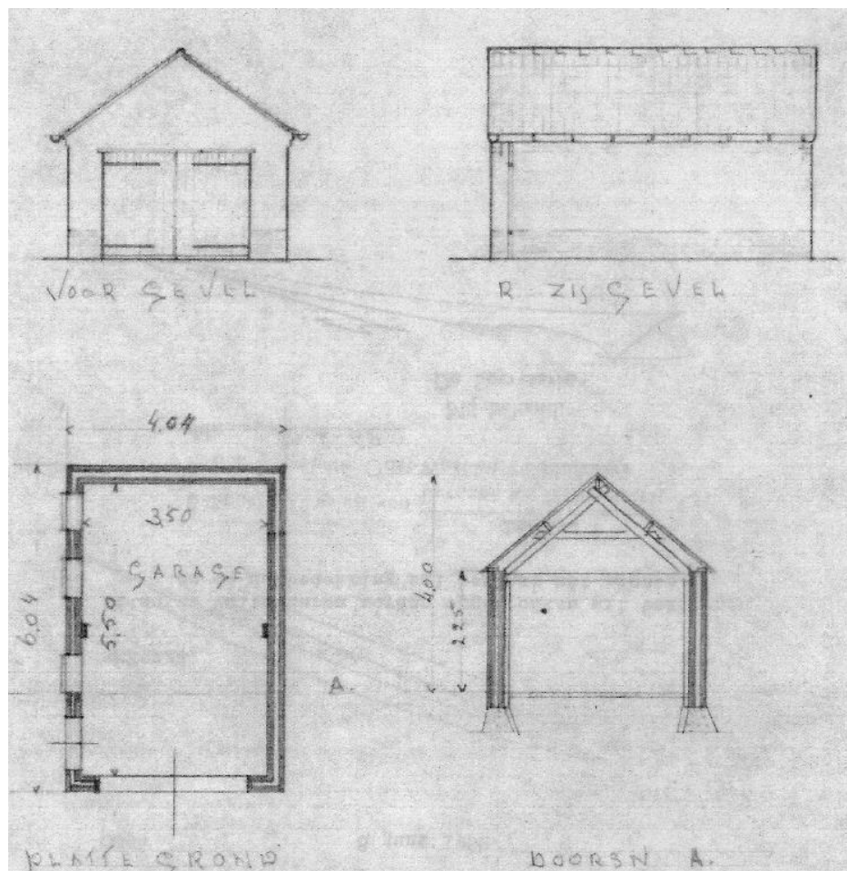
Een voor de bouw van een garage door J. v. G. in 1962 gemaakte tekening voor de weduwe mevrouw Van Roosmalen.
