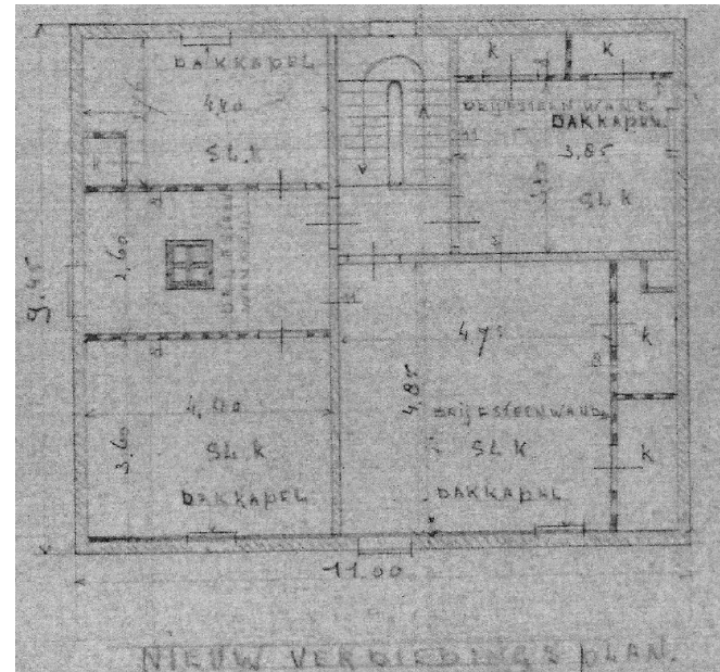
Tekening uit 1955 nieuwe toestand gevel en zolder.
