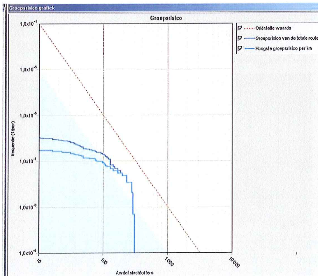
Figuur 4a: Groepsrisico spoortracé Eindhoven – Venlo 2006
