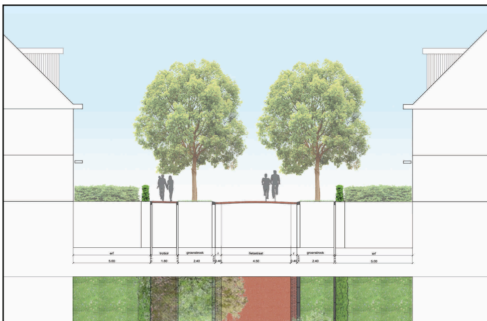
Profiel Opwettenseweg
