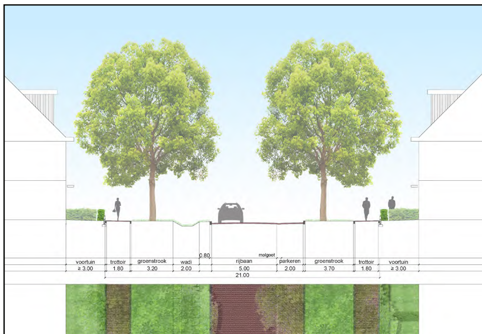
Profiel Dorpslaan
