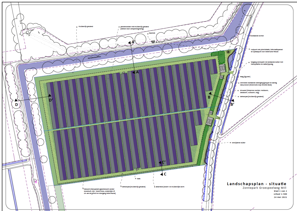
Figuur 5: Opzet zonneveld (blauwe stippellijn is de scheidingslijn Vloet Beheer BV - Gemeenten)
