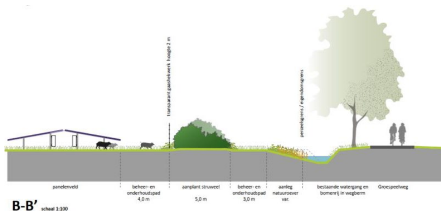
Figuur 6: Dwarsprofiel zijaanzicht zonneveld Groespeelweg Profiel B-B'.
