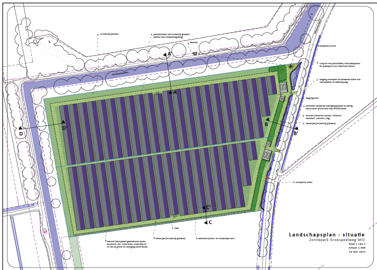
Figuur 10: landschappelijke inpassing plangebied
