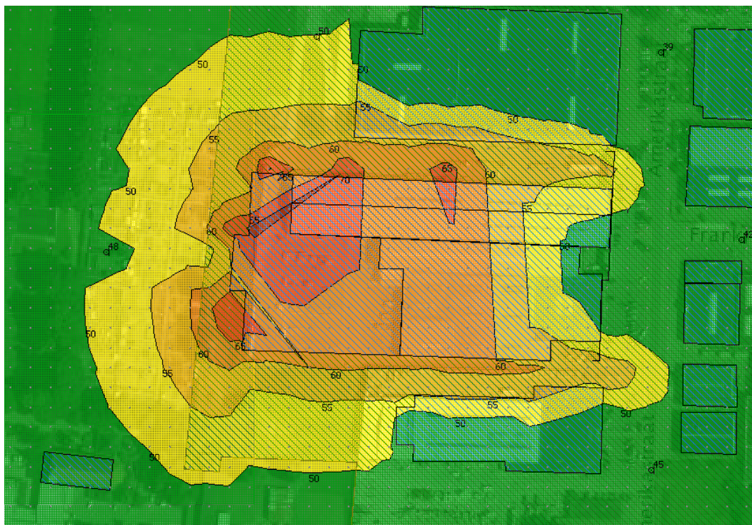
Langtijdgemiddelde geluidbelasting rond bedrijfsperceel Amerikastraat 12, de 50 dB(A)-contour is de grens van het gele vlak
