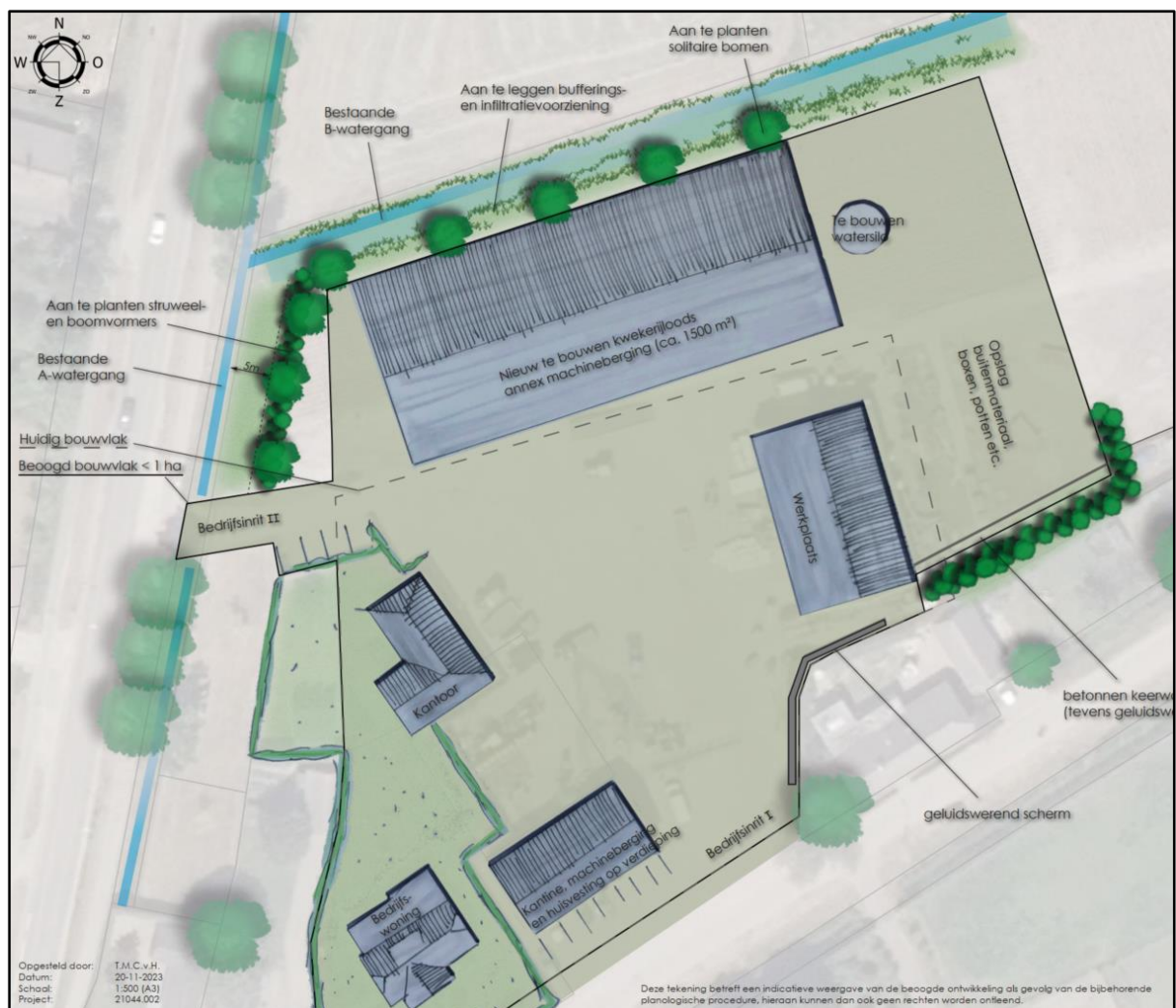
Afbeelding 4: Situatietekening beoogde situatie
