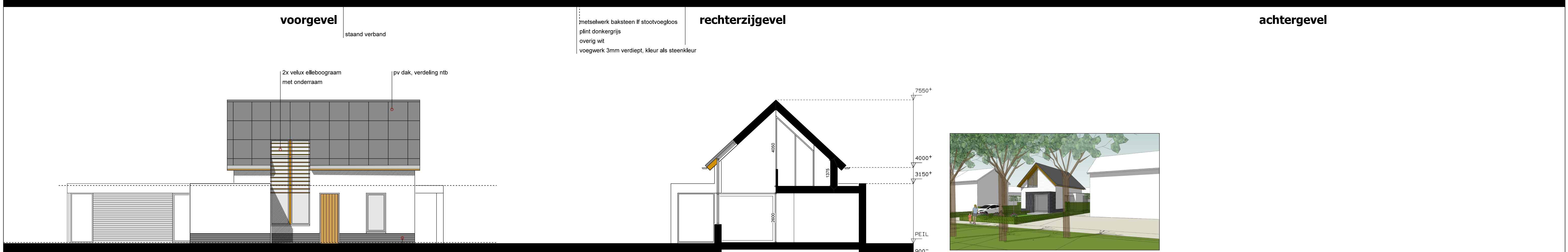
linkerzijgevel
