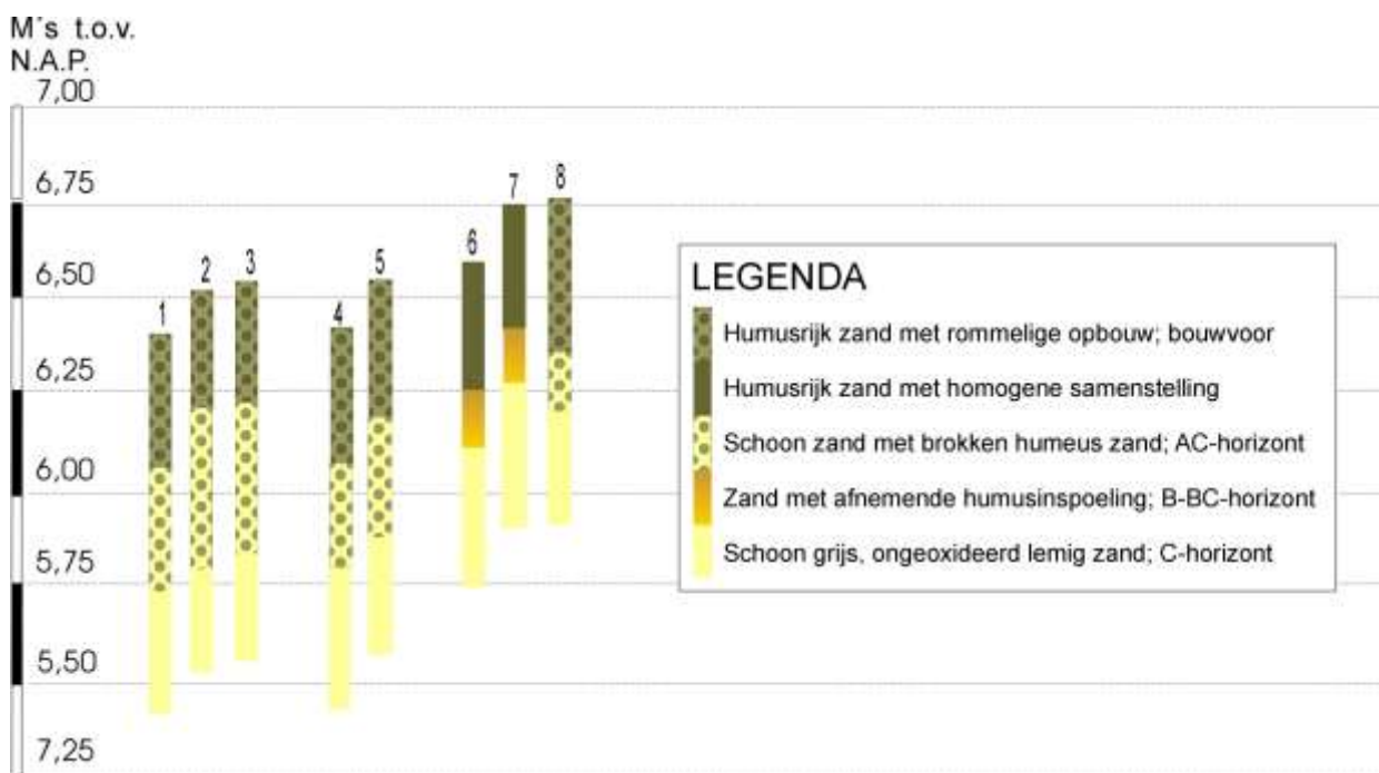
Figuur 24: Boorprofielen
