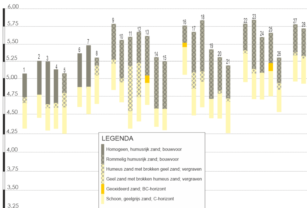
Figuur 25: Boorprofielen
