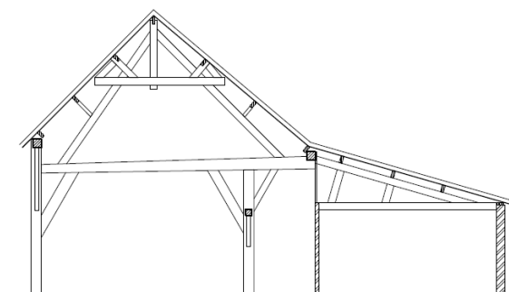
DWARSDOORSNEDE D-D (4e gebint) 0m 5m 10m
