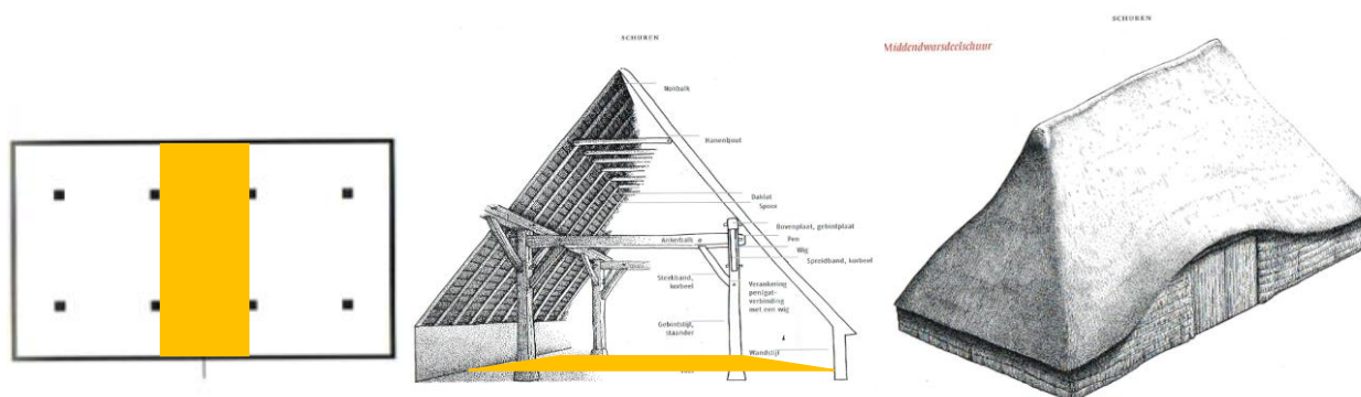
Het principe van een dwarsdeelschuur: plattegrond, impressie constructie en een voorbeeld van een buitenaanzicht met in geel aangegeven de situering van de deel (bron: Erfgoed in de Meierij, Stichting de Brabantse Boerderij)
