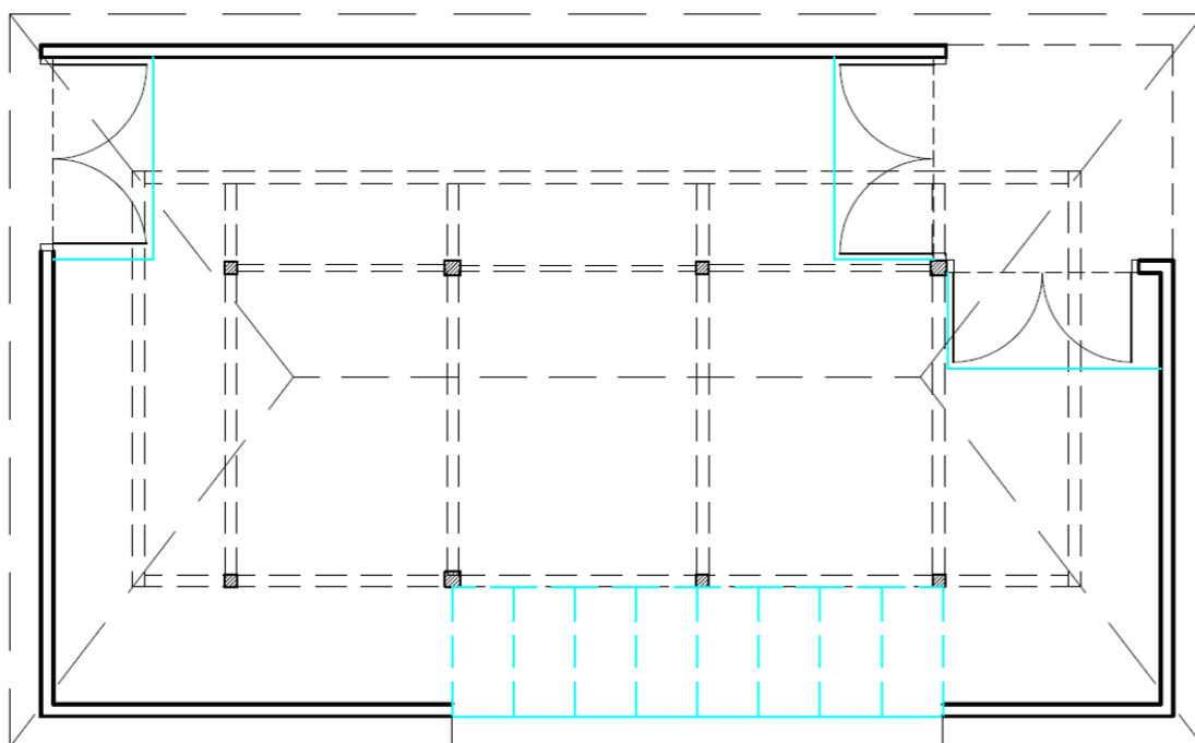
Plattegrond van de schuur zoals deze zou moeten worden, met in blauw ingetekend de locatie's van de glazen puin.
