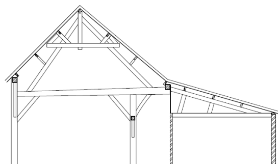
DWARSDOORSNEDE B-B (2e gebint) 0m 5m 10m
