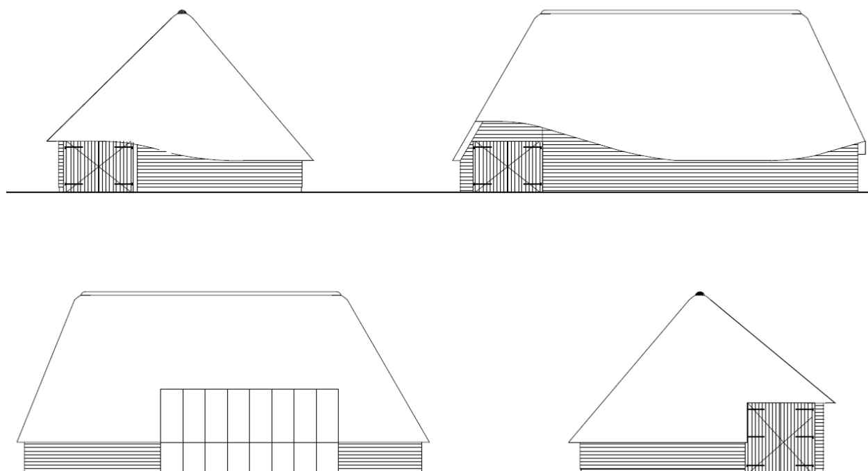
Gevelaanzichten van de schuur na reconstructie: achtereenvolgens: achtergevel (pad-zijde) – rechter zijgevel (straatzijde) – voorgevel (boerderijzijde) – linker zijgevel (veldzijde)
