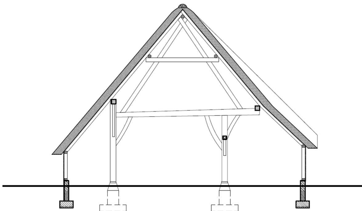
Doorsnede van de nieuwe situatie met de vorm zoals deze oorspronkelijk geweest moet zijn. (isolatielagen nog niet ingetekend)
