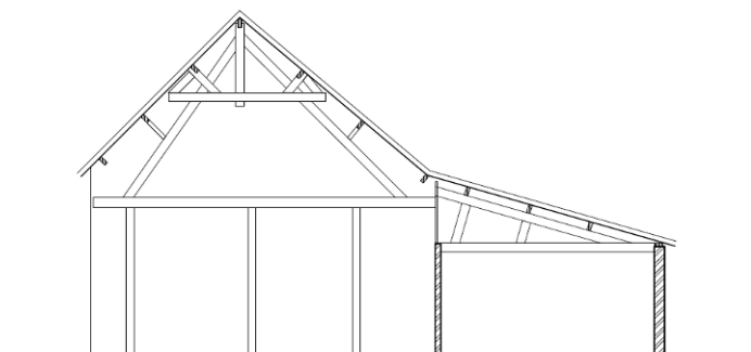
DWARSDOORSNEDE D-D 0m 5m 10m
