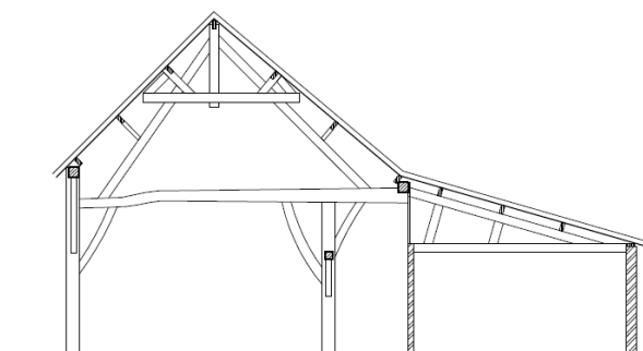
DWARSDOORSNEDE C-C (3e gebint) 0m 5m 10m
