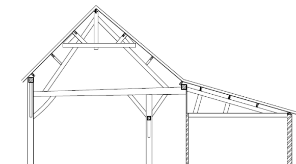
DWARSDOORSNEDE A-A (1e gebint) 0m 5m 10m
