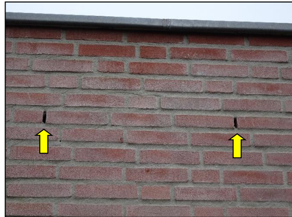
Figuur 11. Toegang voor vleermuizen in de vorm van open stootvoegen aan de achterzijde van Marktstraat 33-37.
