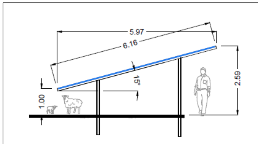
Afbeelding 8: Doorsnede van de basisconstructie
