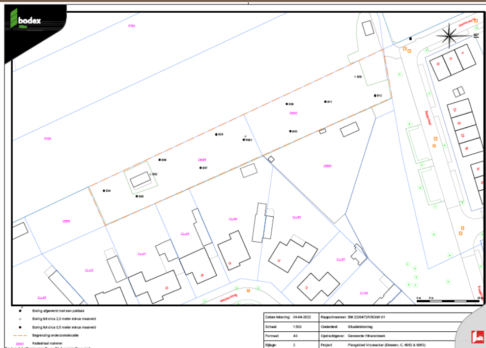
Afbeelding 4: situatietekening met boorpunten (bron tekening: Bodex Milieu)
