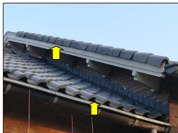
Figuur 13. Ruimtes langs de dakrand bieden toegangsmogelijkheden tot onder het dak.
