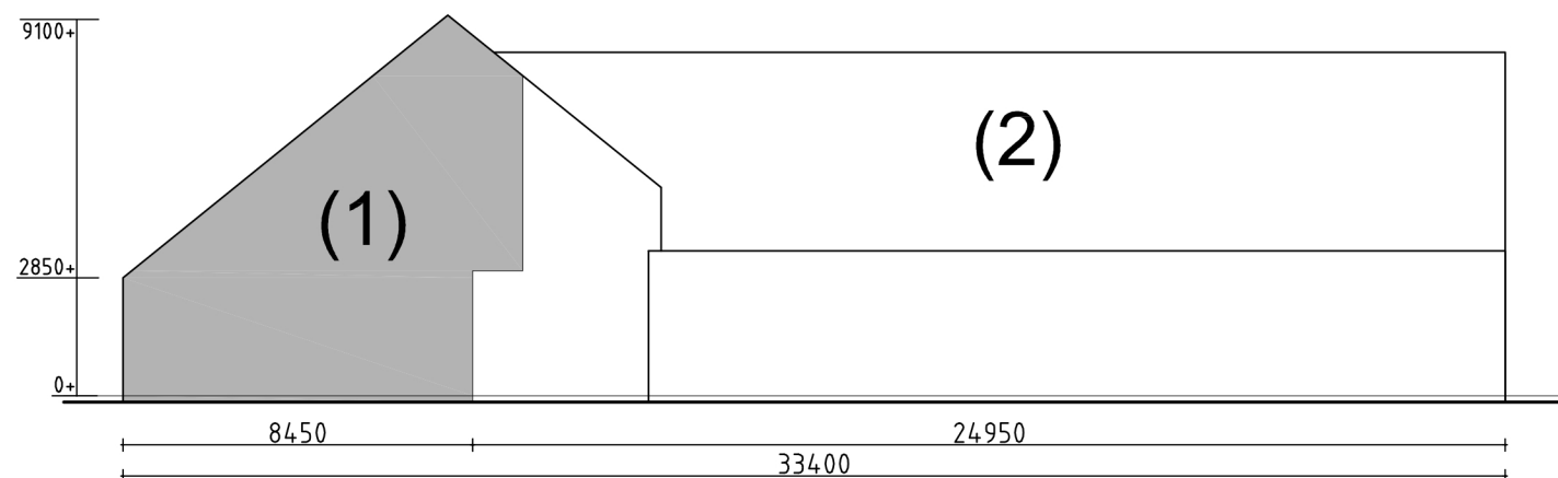
VOORGEVEL
