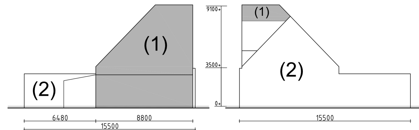
LINKER ZIJGEVEL
