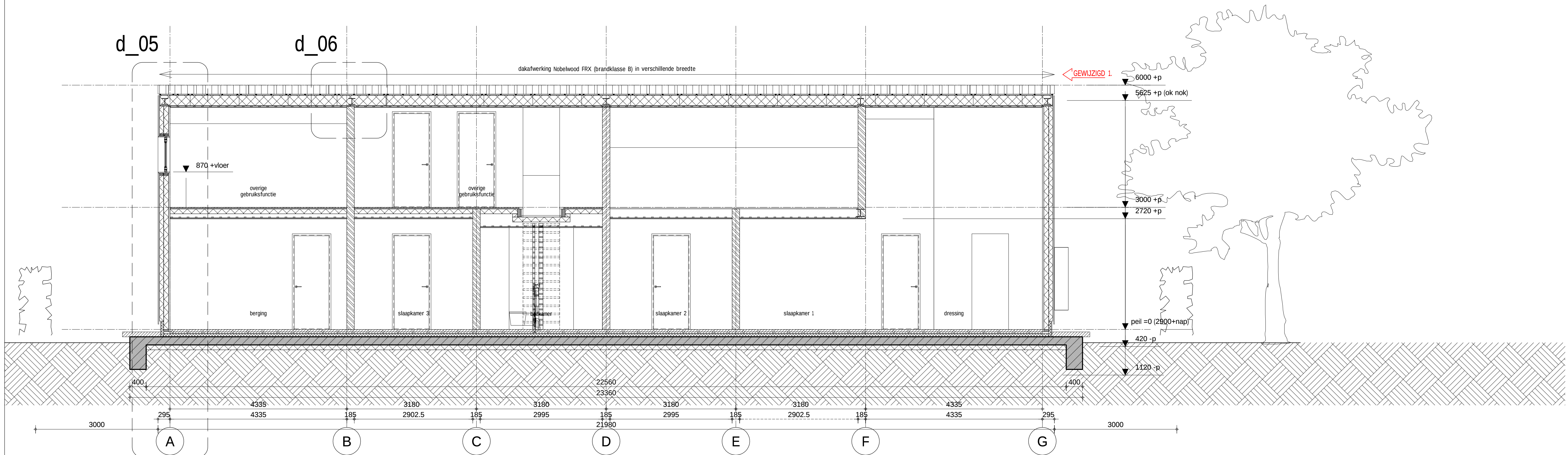
doorsnede -3-
