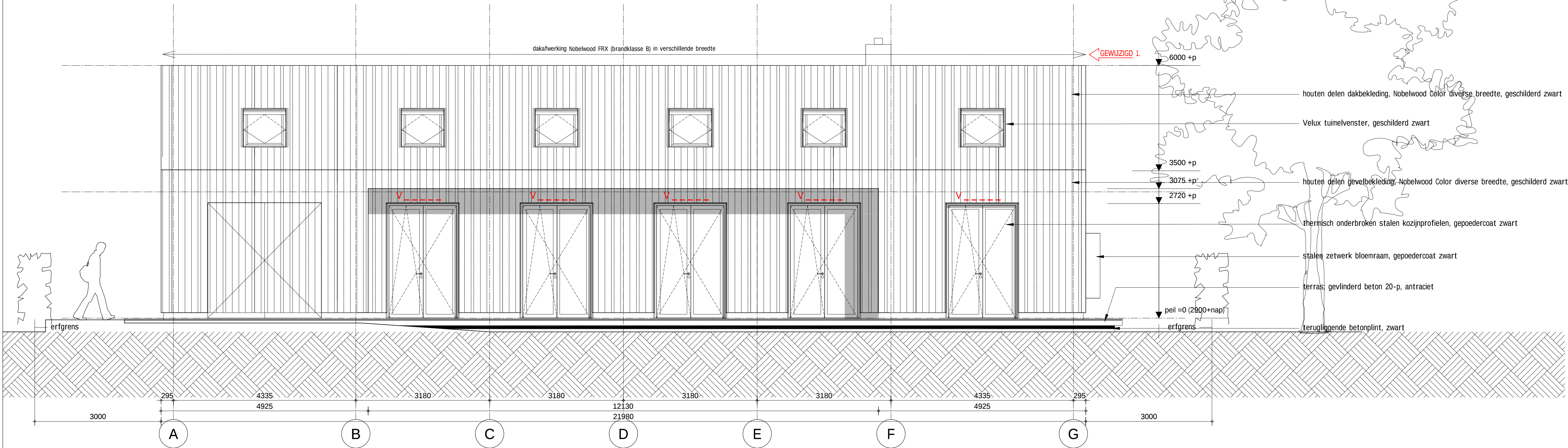
aanzicht noordgevel
