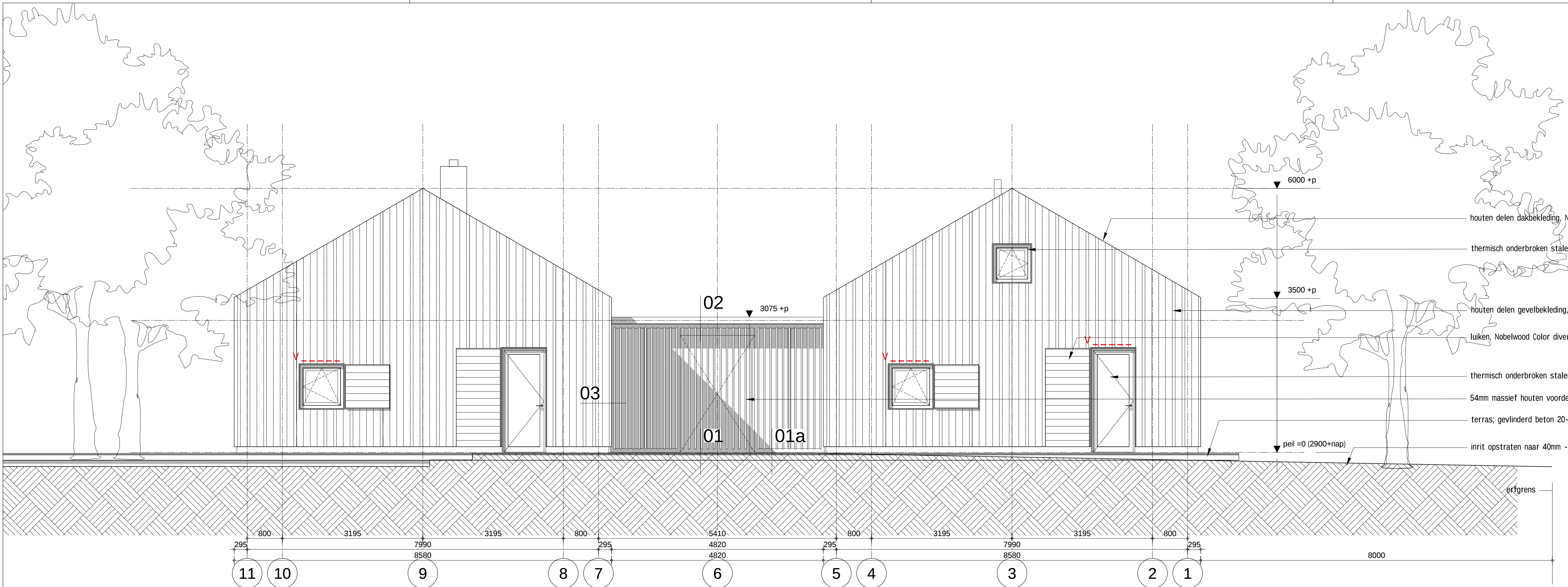
aanzicht oostgevel
