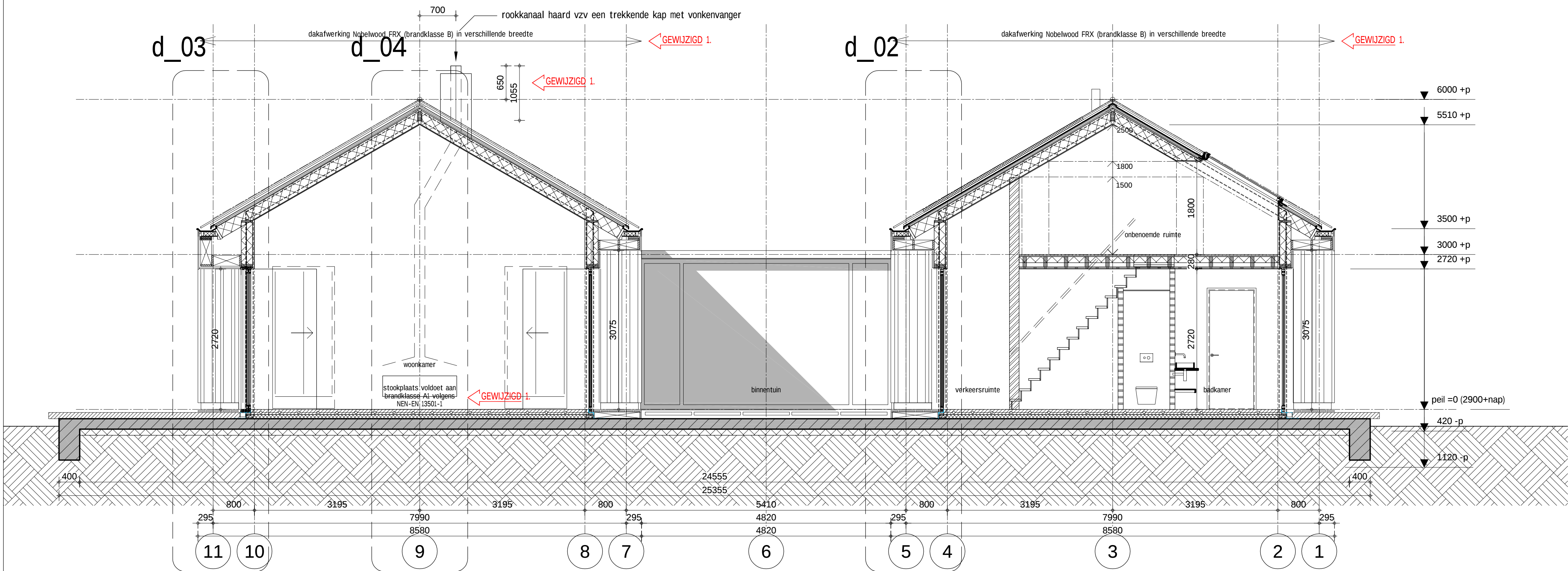
doorsnede -2-
