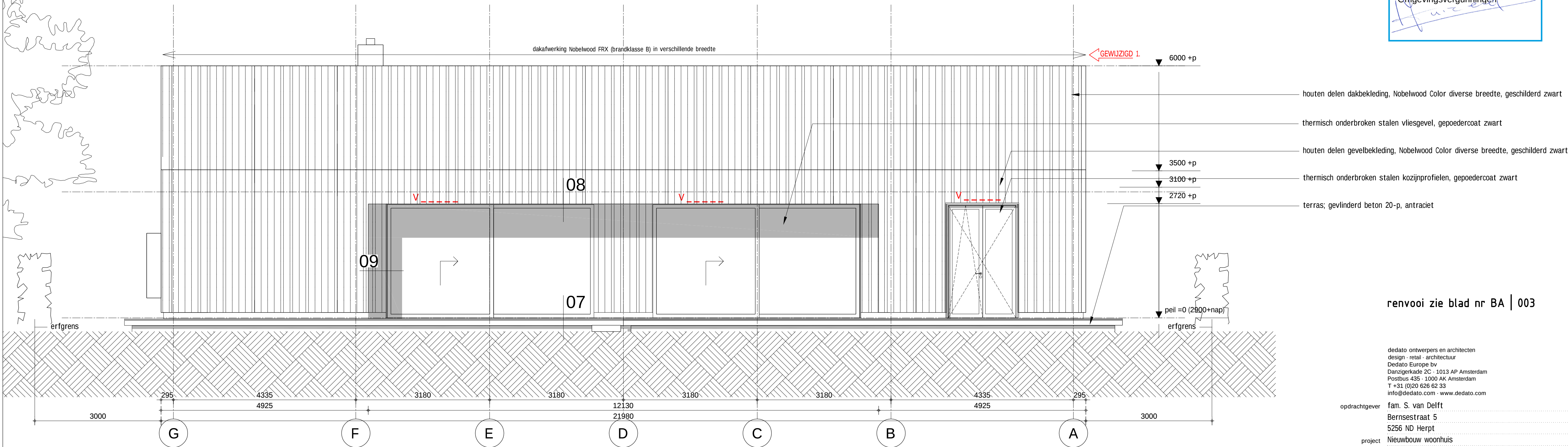
aanzicht zuidgevel
