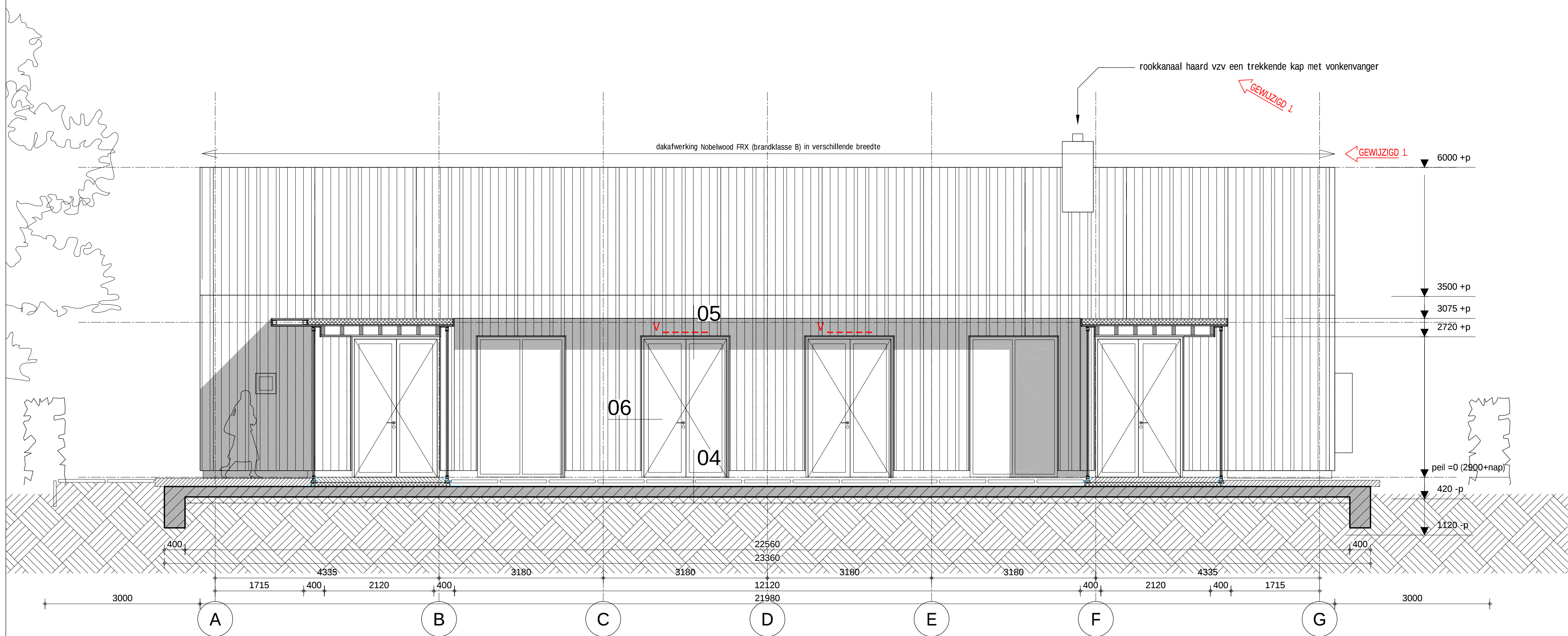
doorsnede -4-
