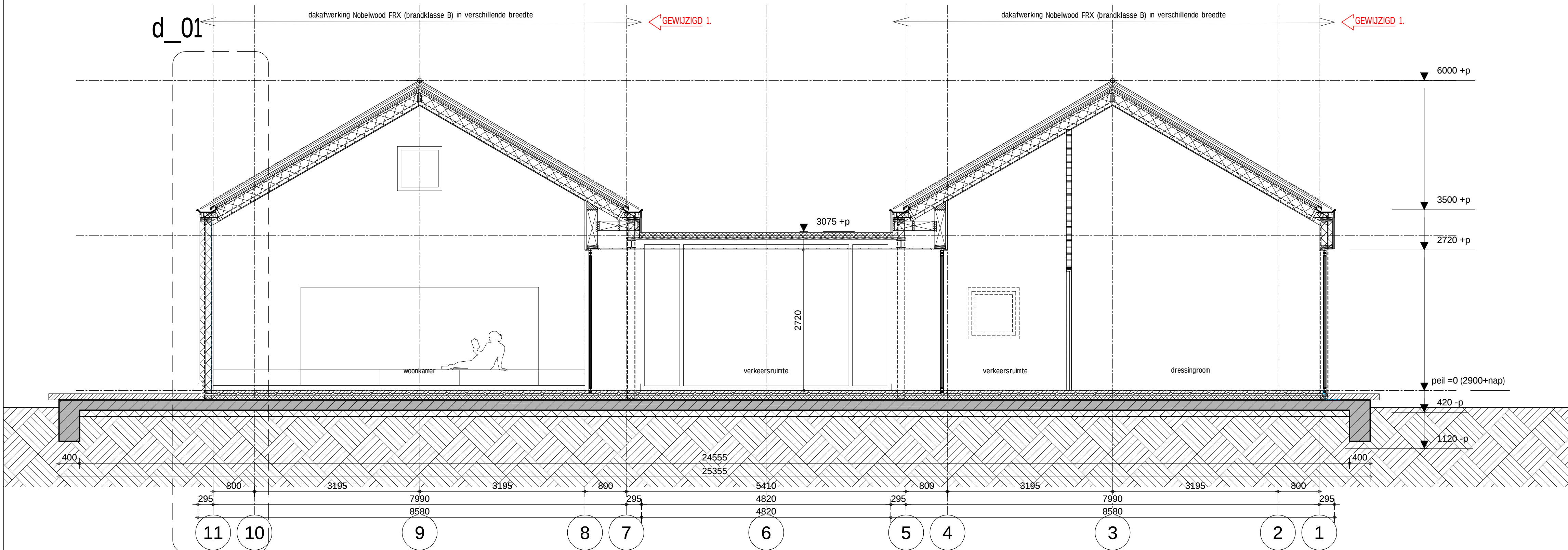
doorsnede -1-
