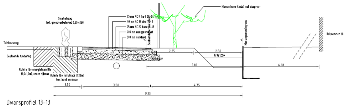
Figuur 2. Dwarsprofiel ter hoogte van Tuinbouwweg 18.
