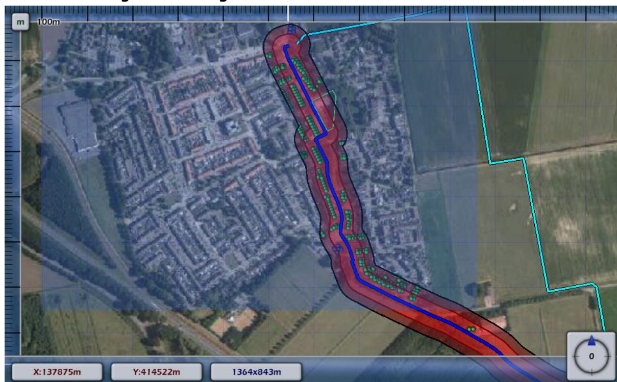
Figuur 4: Huidige ligging invloedsgebied (1% letaliteit) van de hogedruk aardgasleiding Z-517-04. De binnenste contour is de 100% letaliteitsafstand.
