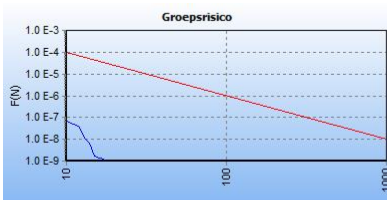
Figuur 6: FN curve behorend bij de boven aangegeven kilometer leiding.
