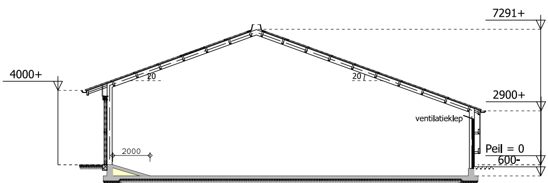
DOORSNEDE GEBOUW 3
