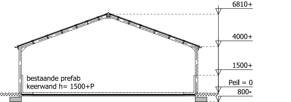
DOORSNEDE GEBOUW 4
