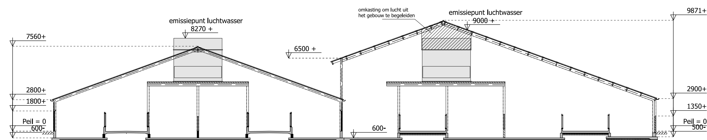
DOORSNEDE GEBOUW 2
