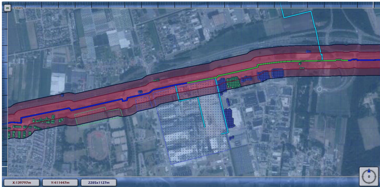
Figuur 7: Kilometer leiding met het hoogste groepsrisico (groen). In het blauw is de gehele leiding aangegeven. De rode contour hieromheen is het invloedsgebied van de leiding.
