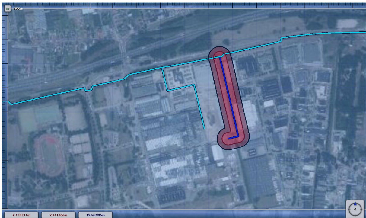
Figuur 5: Huidige ligging invloedsgebied (1% letaliteit) van de hogedruk aardgasleiding Z-517-16. De binnenste contour is de 100% letaliteitsafstand.
