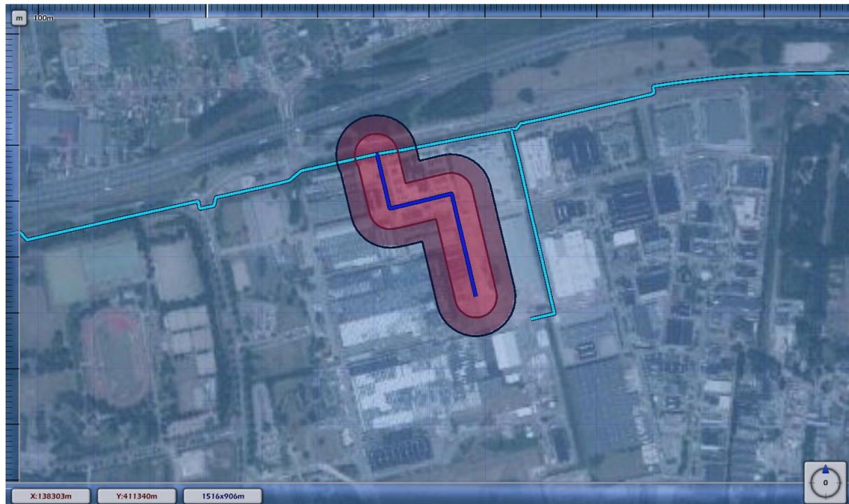
Figuur 6: Huidige ligging invloedsgebied (1% letaliteit) van de hogedruk aardgasleiding Z-517-06. De binnenste contour is de 100% letaliteitsafstand.
