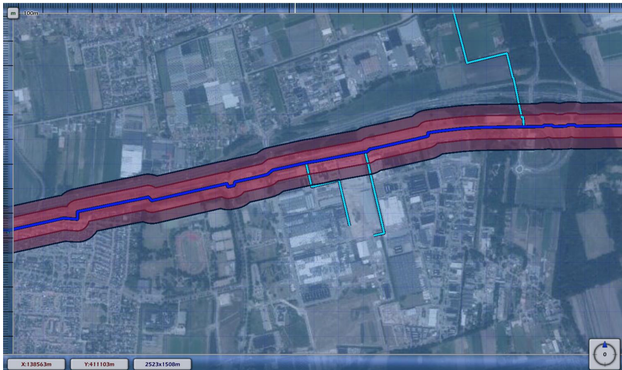
Figuur 4: Huidige ligging invloedsgebied (1% letaliteit) van de hogedruk aardgasleiding Z-517-12. De binnenste contour is de 100% letaliteitsafstand.
