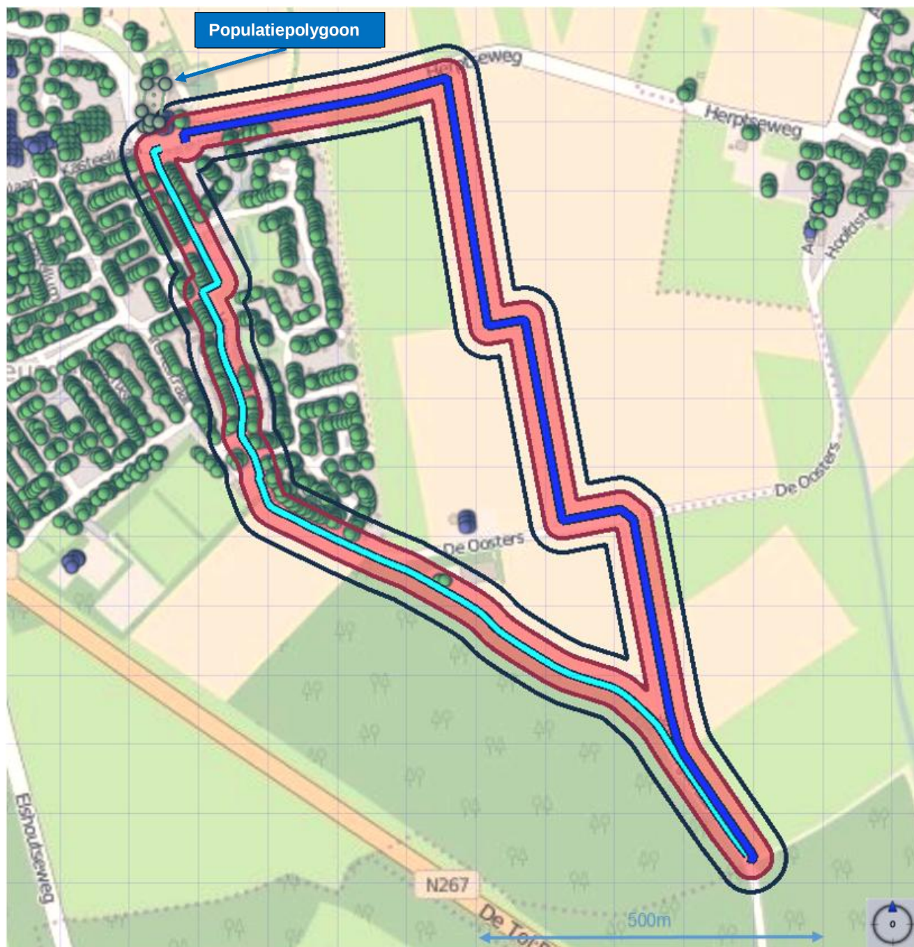
Figuur 2 Invloedsgebied van de leiding Z-517-04. De zwarte lijn geeft het invloedsgebied (1% letaliteitsgrens) van de leiding weer; het rode gebied geeft de 100% letaliteitsgrens weer. De lichtblauwe leiding geeft de huidige situatie weer, de donkerblauwe leiding de toekomstige situatie.
