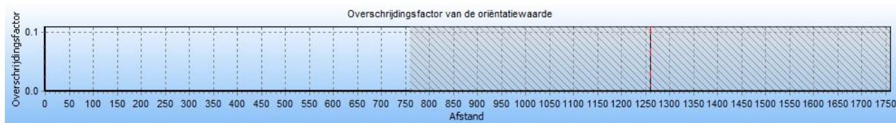
Figuur 7 Overschrijding van het groepsrisico als functie van de stationing van de Z-517-04.
