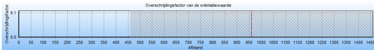
Figuur 5 Overschrijding van het groepsrisico als functie van de stationing van de Z-517-04.
