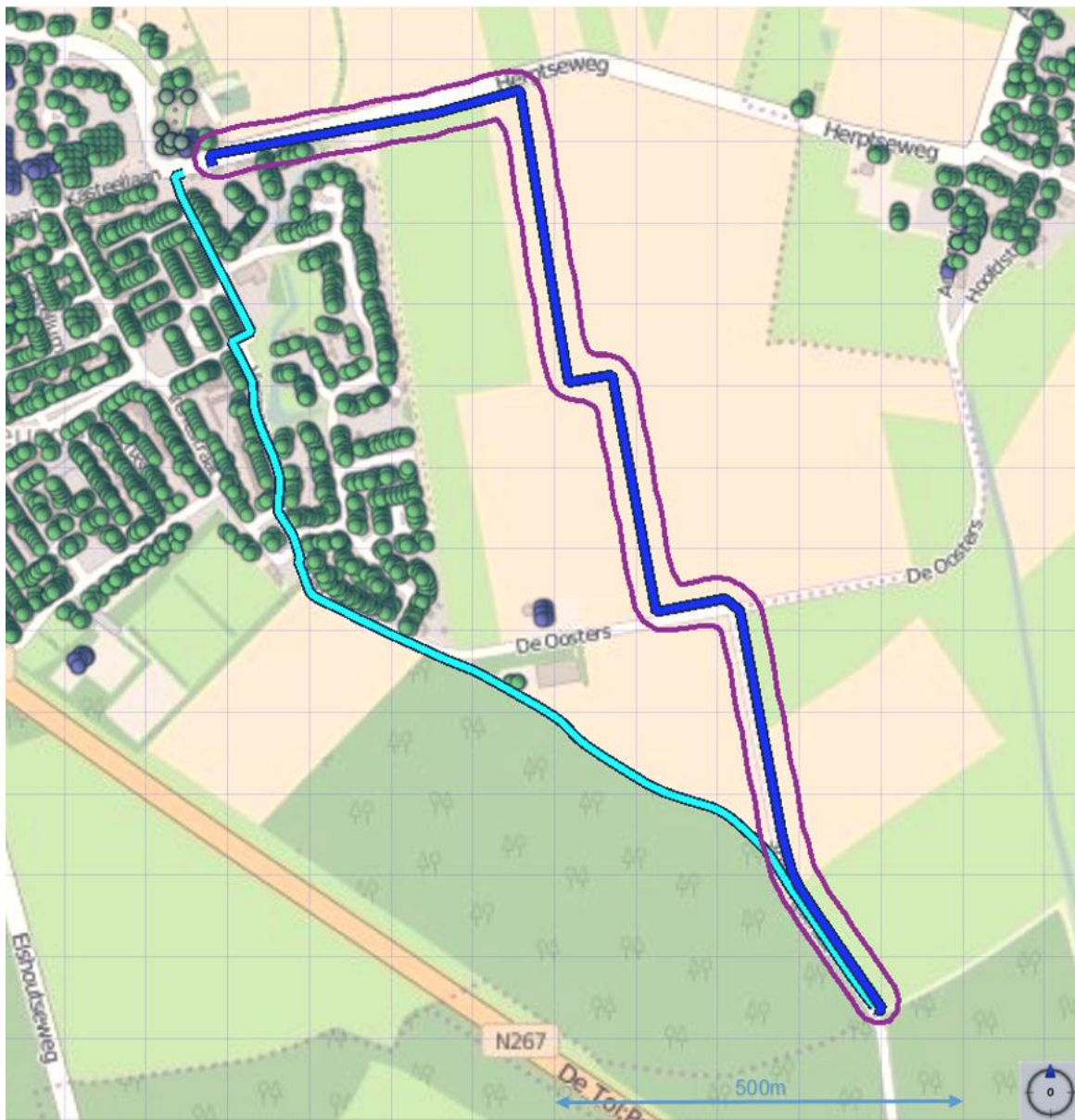
Figuur 4 Ligging van gastransportleiding Z-517-04 (donkerblauw) in de toekomstige situatie. De plaatsgebonden risicocontouren rondom de leiding zijn, wanneer aanwezig, weergegeven met de volgende kleuren:
