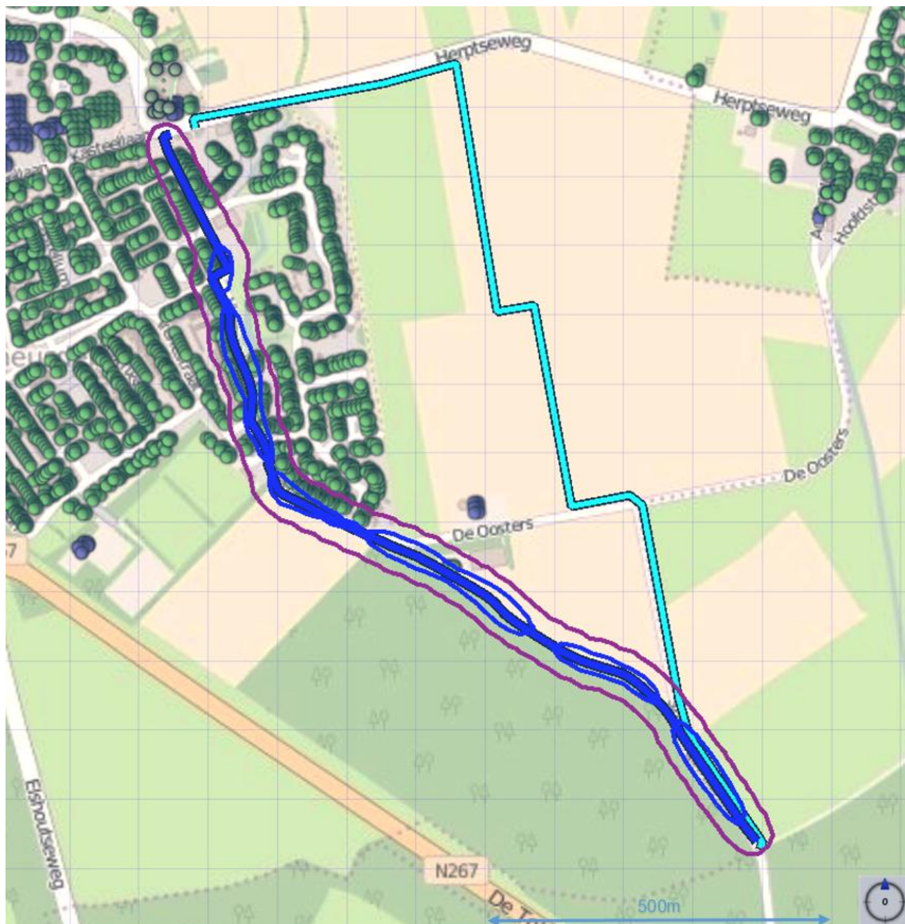
Figuur 3 Ligging van gastransportleiding Z-517-04 (donkerblauw) in de huidige situatie. De plaatsgebonden risicocontouren rondom de leiding zijn, wanneer aanwezig, weergegeven met de volgende kleuren:
