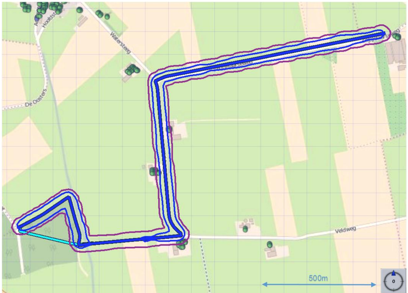
Figuur 3 Ligging van gastransportleiding Z-517-05 (donkerblauw) in de huidige situatie. De plaatsgebonden risicocontouren rondom de leiding zijn, wanneer aanwezig, weergegeven met de volgende kleuren:
