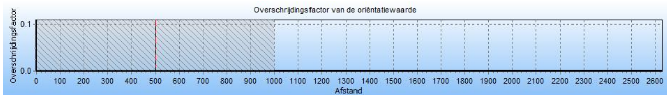
Figuur 5 Overschrijding van het groepsrisico als functie van de stationing van de Z-517-05.
