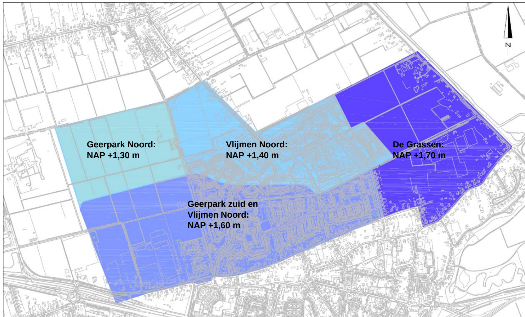
Figuur 4: Beoogde waterpeilen en peilvakken
