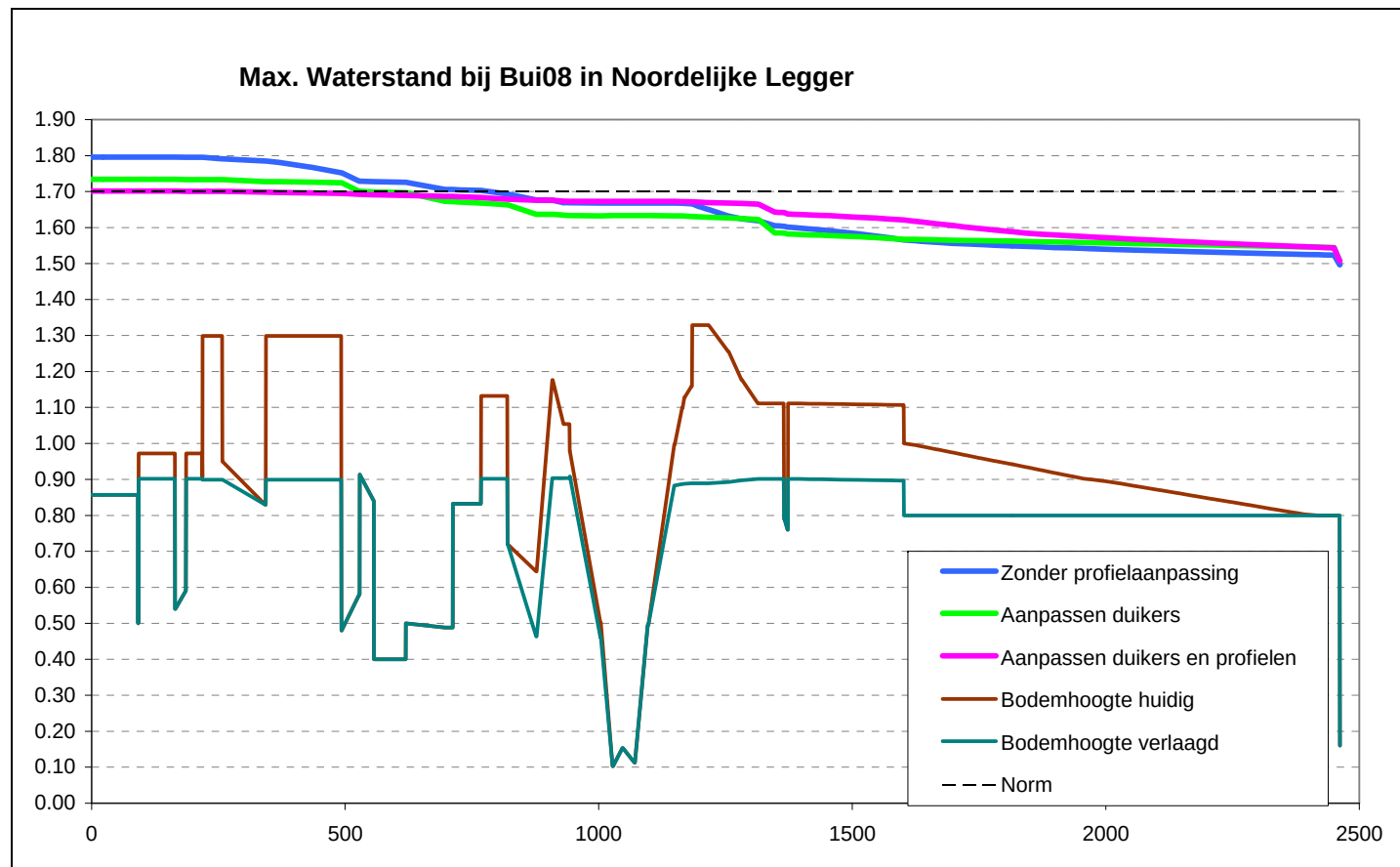
Figuur 10: Lengteprofiel noordelijke leggerwatergang met bodemhoogtes en maximale waterstanden (m NAP) voor verschillende situaties in fase 2; het voorkomen van verdrinken van riooldrempels is alleen mogelijk door het verdiepen van de watergang tot minimaal NAP +0,90 m en het verruimen van duikers 5
