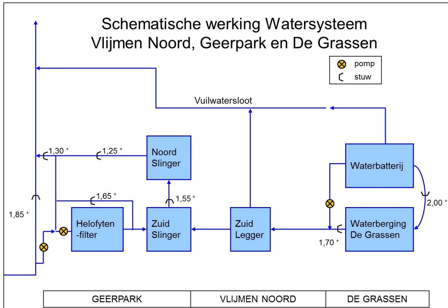
Figuur 11: Schematisatie werking watersysteem Vlijmen Noord (eindsituatie met de uitgangspunten zoals toegepast voor het effect op de waterberging en de waterbalans in paragraaf 4.3.3 en 4.3.4.)
