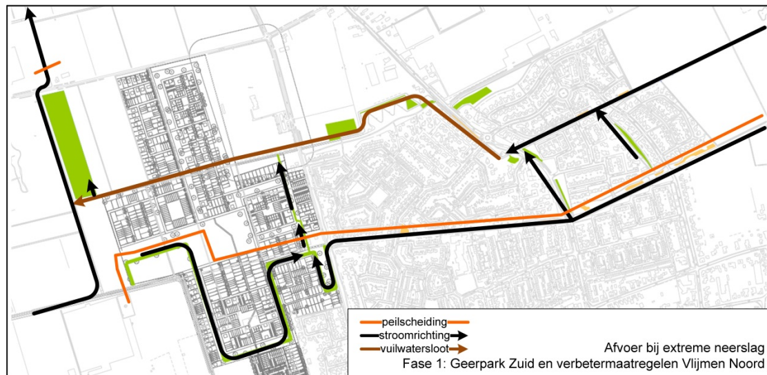
Figuur 5b: Afvoer bij extreme neerslag (fase 1)
