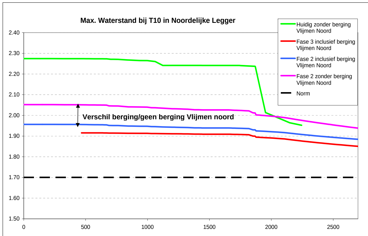
Figuur 8: Lengteprofiel noordelijke leggerwatergang met maximale waterstanden (m NAP) voor verschillende situaties; berging in Vlijmen Noord geeft positief effect op waterstanden 3
