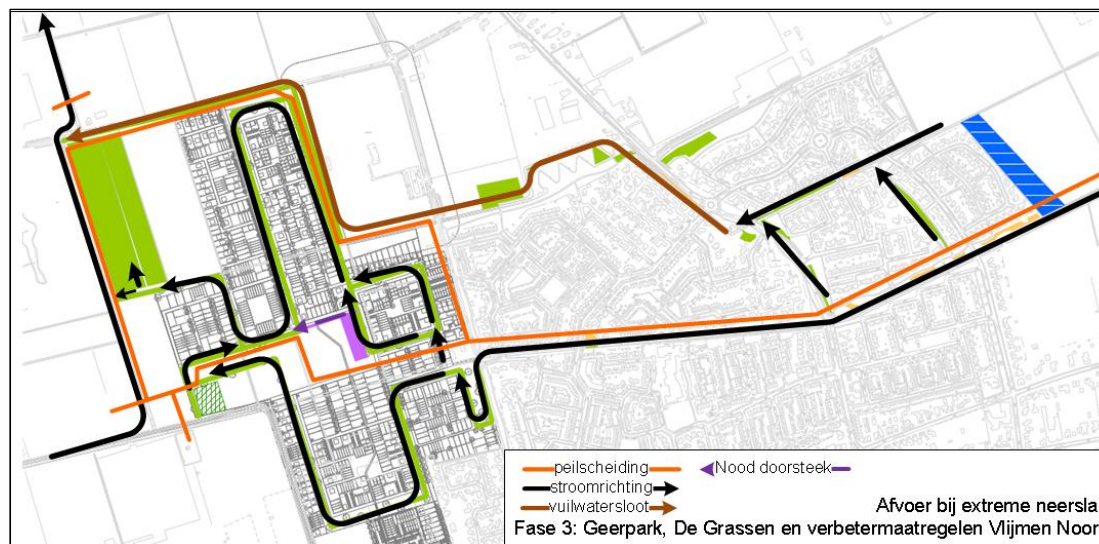
Figuur 7b: Afvoer bij extreme neerslag (fase 3)
