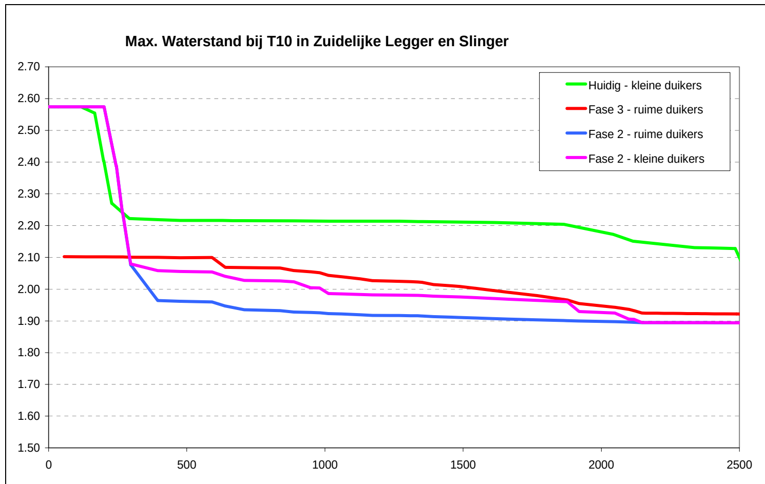
Figuur 9: Lengteprofiel zuidelijke leggerwatergang met maximale waterstanden (m NAP) voor verschillende situaties; verruimen van duikers is pas vanaf fase 3 noodzakelijk 4
