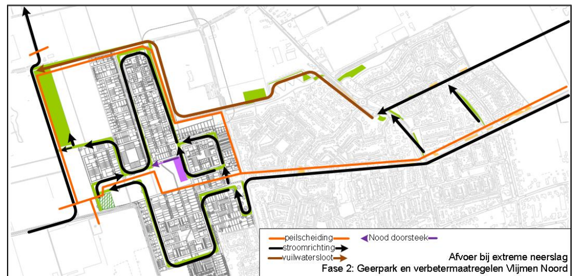
Figuur 6b: Afvoer bij extreme neerslag (fase 2)
