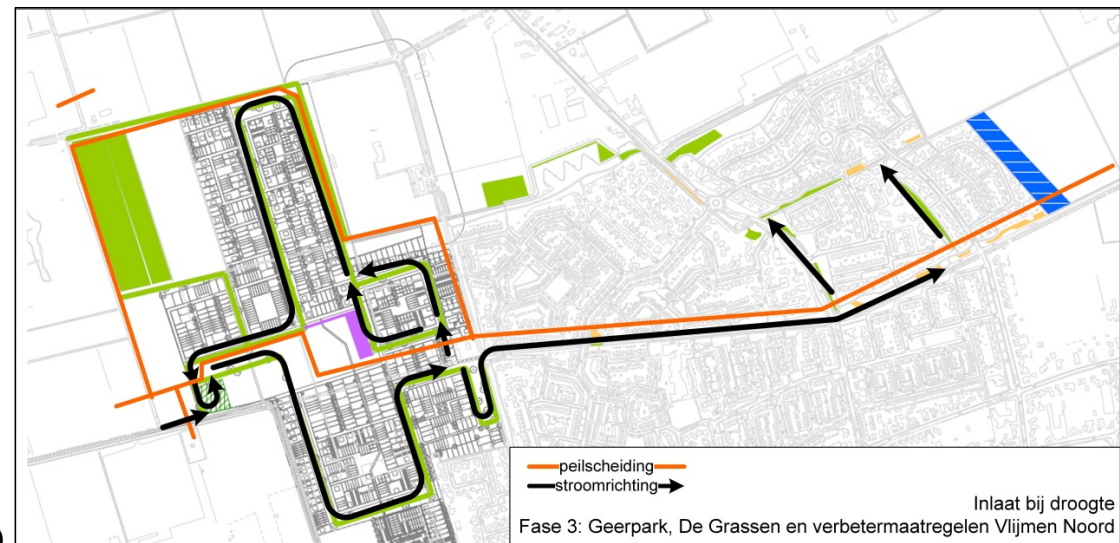
Figuur 7c: Inlaat bij droogte (fase 3)
