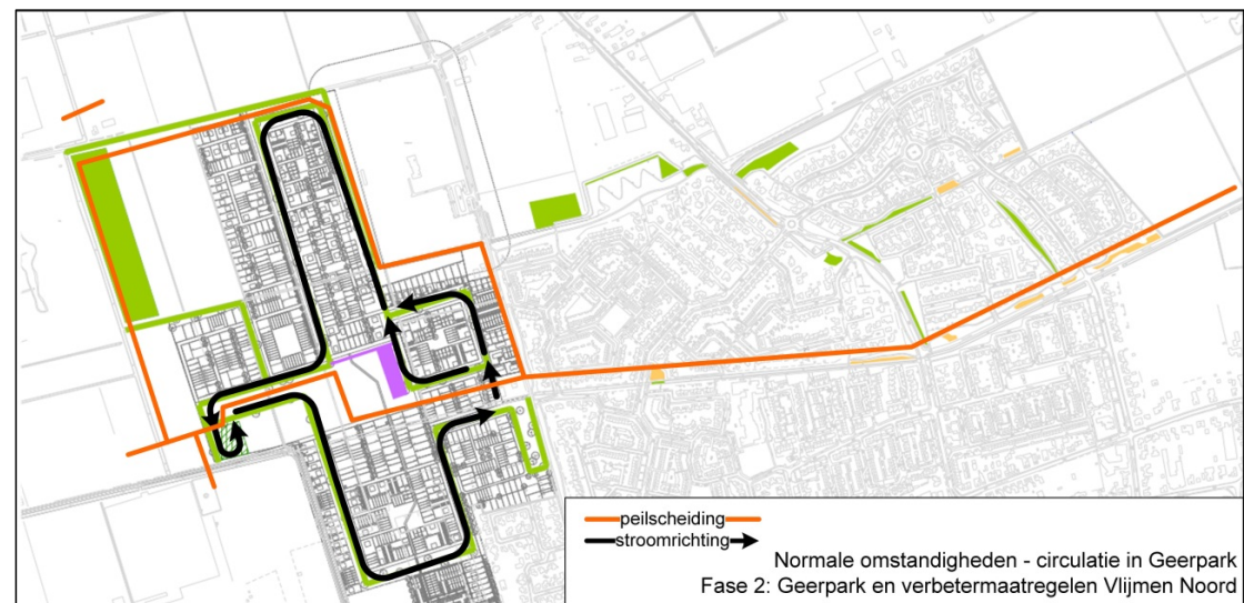
Figuur 6a: Normale omstandigheden (fase 2)
