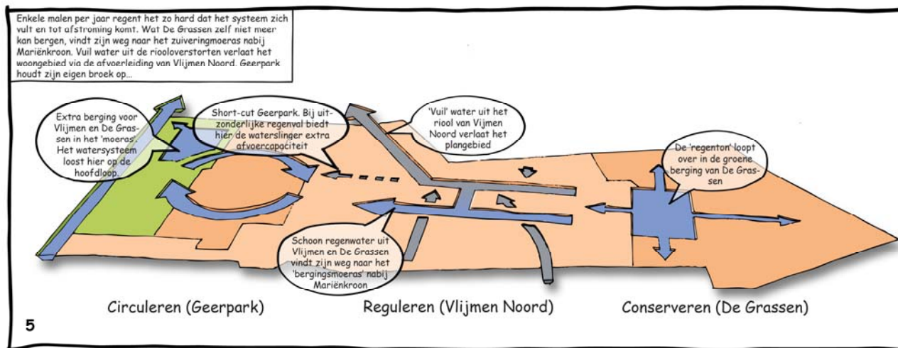
Figuur 3.5: Watersysteem werking toekomstig watersysteem onder natte omstandigheden
