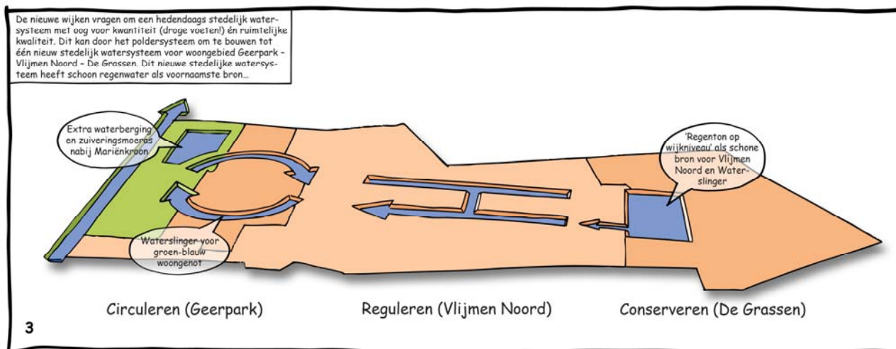
Figuur 3.3: Watersysteem werking toekomstig watersysteem onder normale omstandigheden
