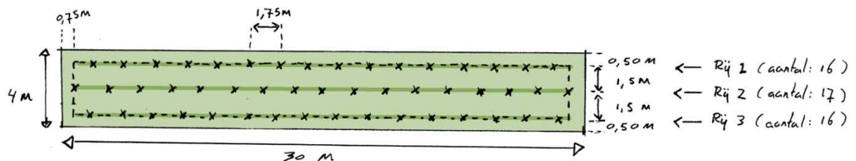
Afbeelding 3. Schets plantvak struiklaag zijde A59 en ter hoogte van het bedrijfsgebouw, in driehoeksverband (1,75 m).
