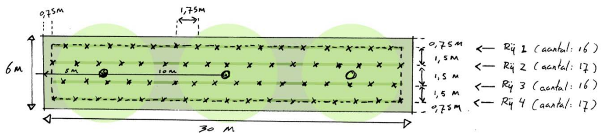
Afbeelding 2. Schets plantvak bomenrij met struiklaag, in driehoeksverband (1,75 m).
