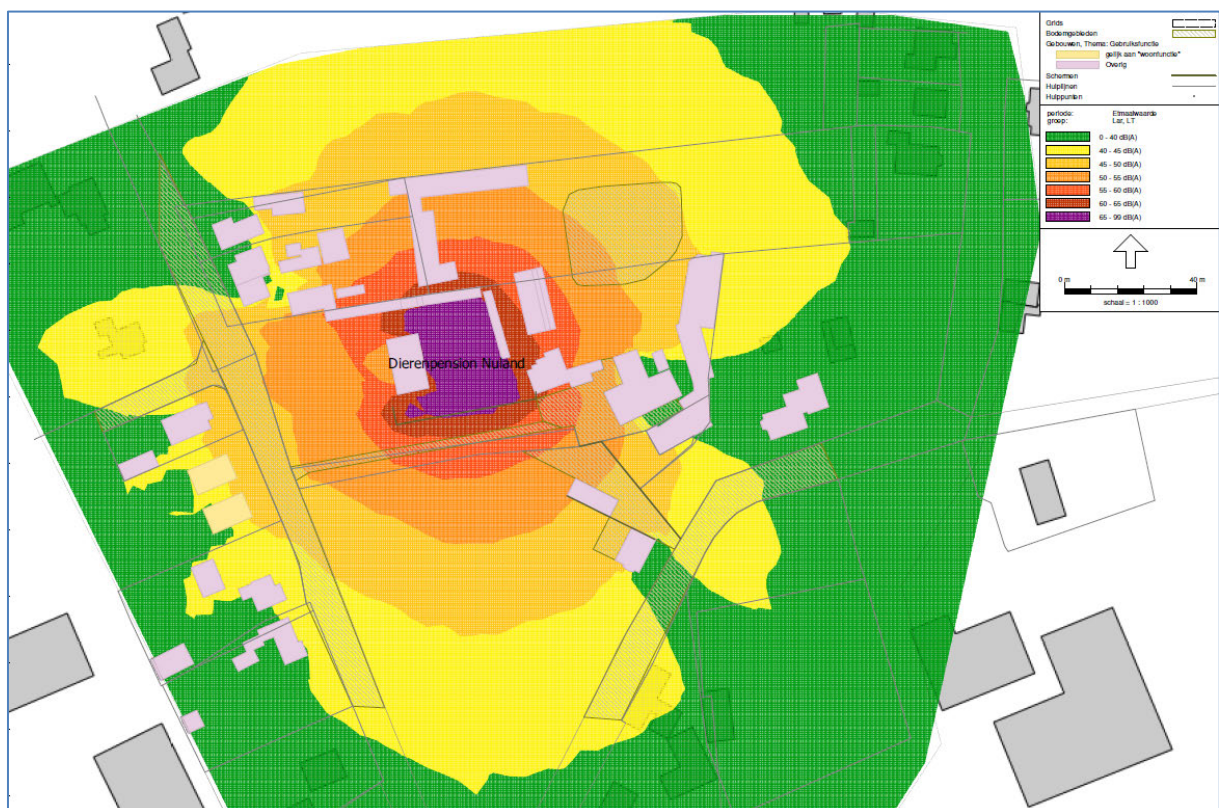
Afbeelding 4. Geluidcontour op hoogte 4,0 meter
