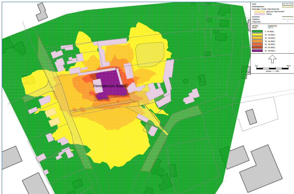
Afbeelding 3. Geluidcontour op hoogte 1,5 meter
