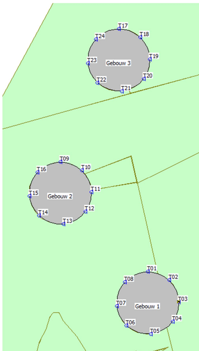
Afbeelding 4 Ligging rekenpunten
