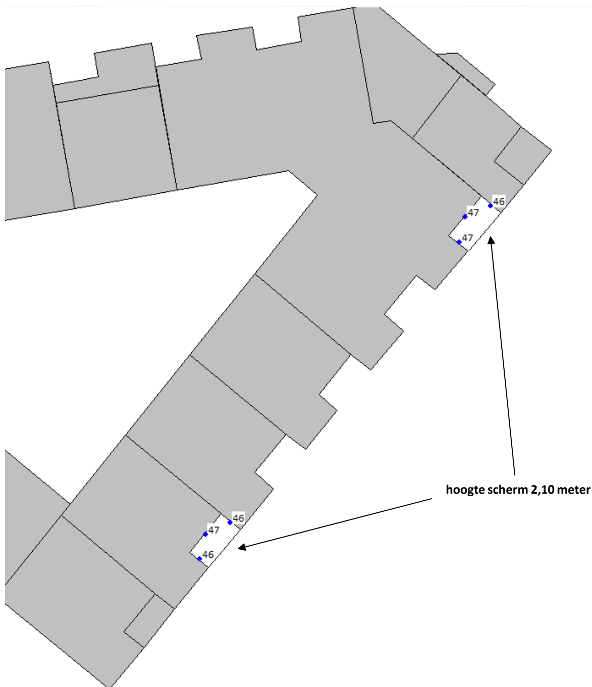
Figuur 1-1 Geluidsbelasting achterliggende gevel (incl. aftrek) begane grond
