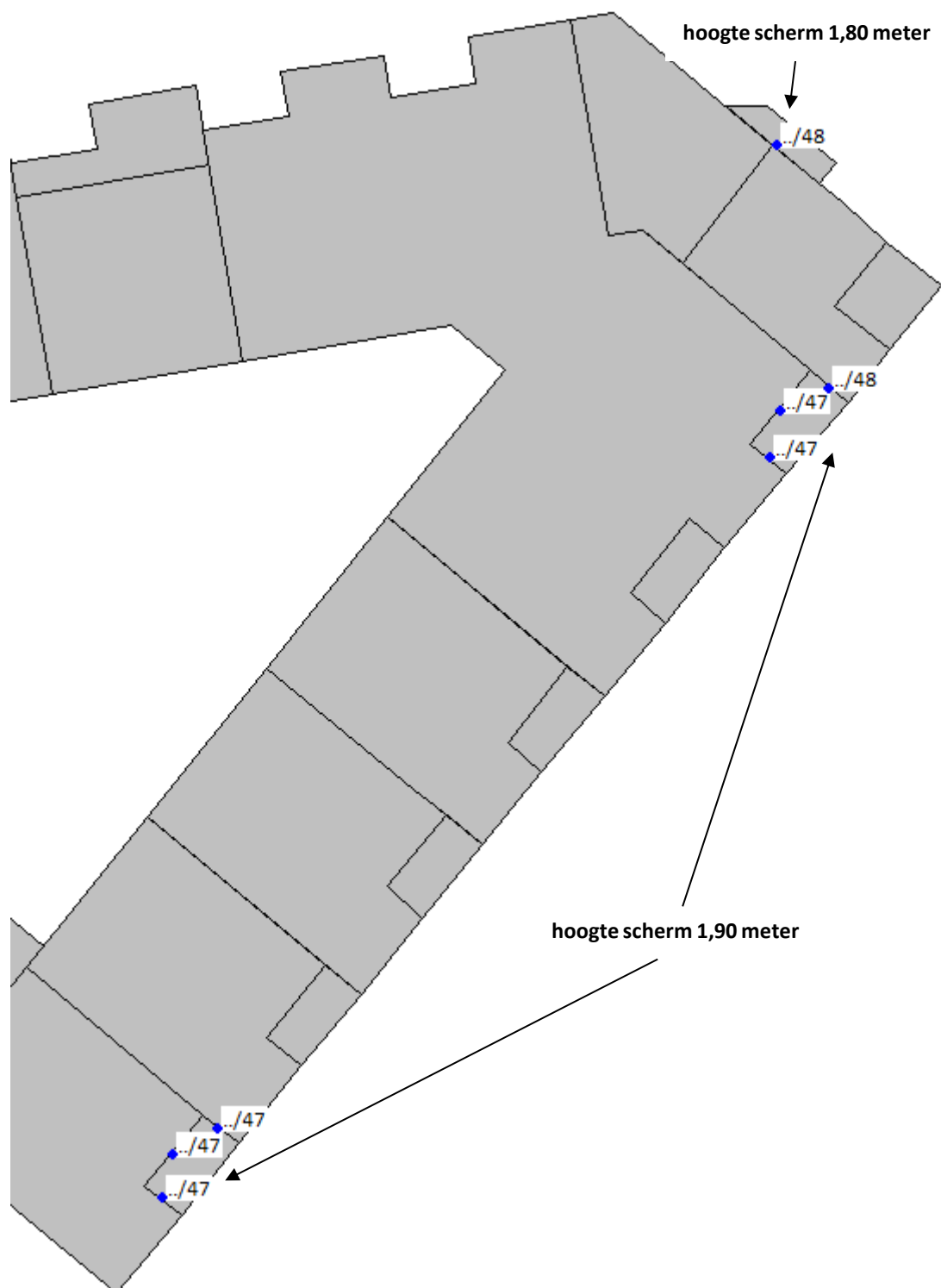
Figuur 1-2 Geluidsbelasting achterliggende gevel (incl. aftrek) 1 e verdieping
