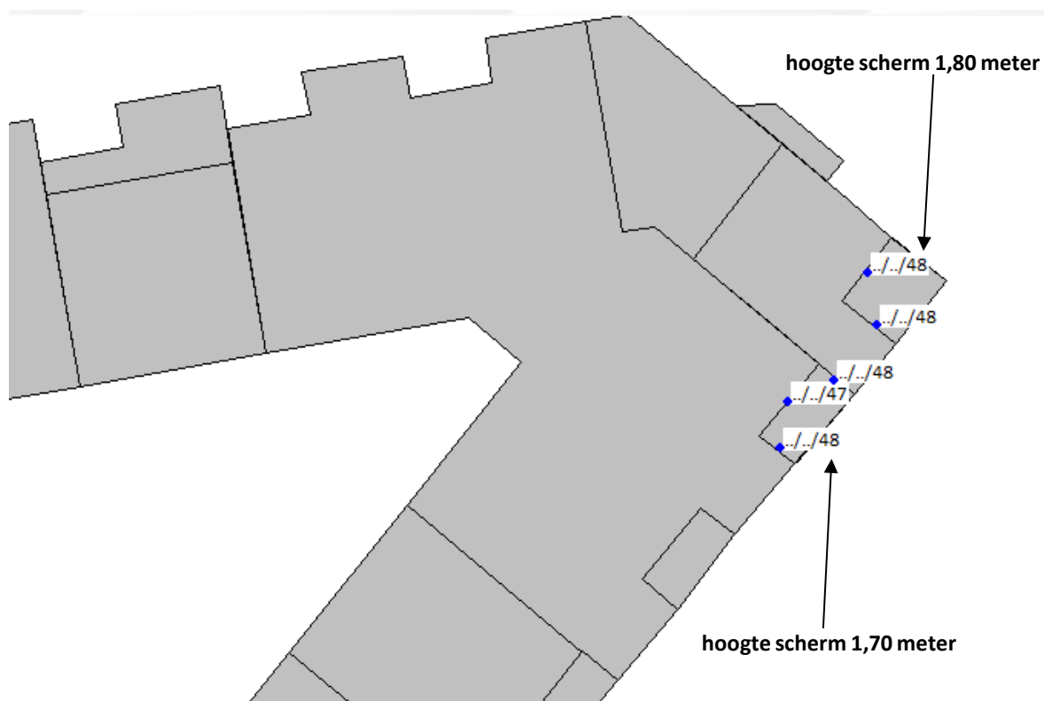
Figuur 1-3 Geluidsbelasting achterliggende gevel (incl. aftrek) 2e verdieping
