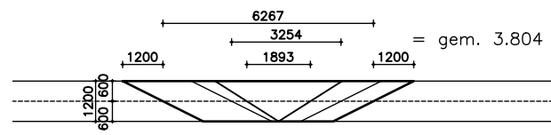
Dwarsdoorsnede Wadi
