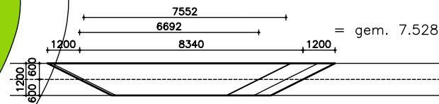
Langdoorsnede Wadi
