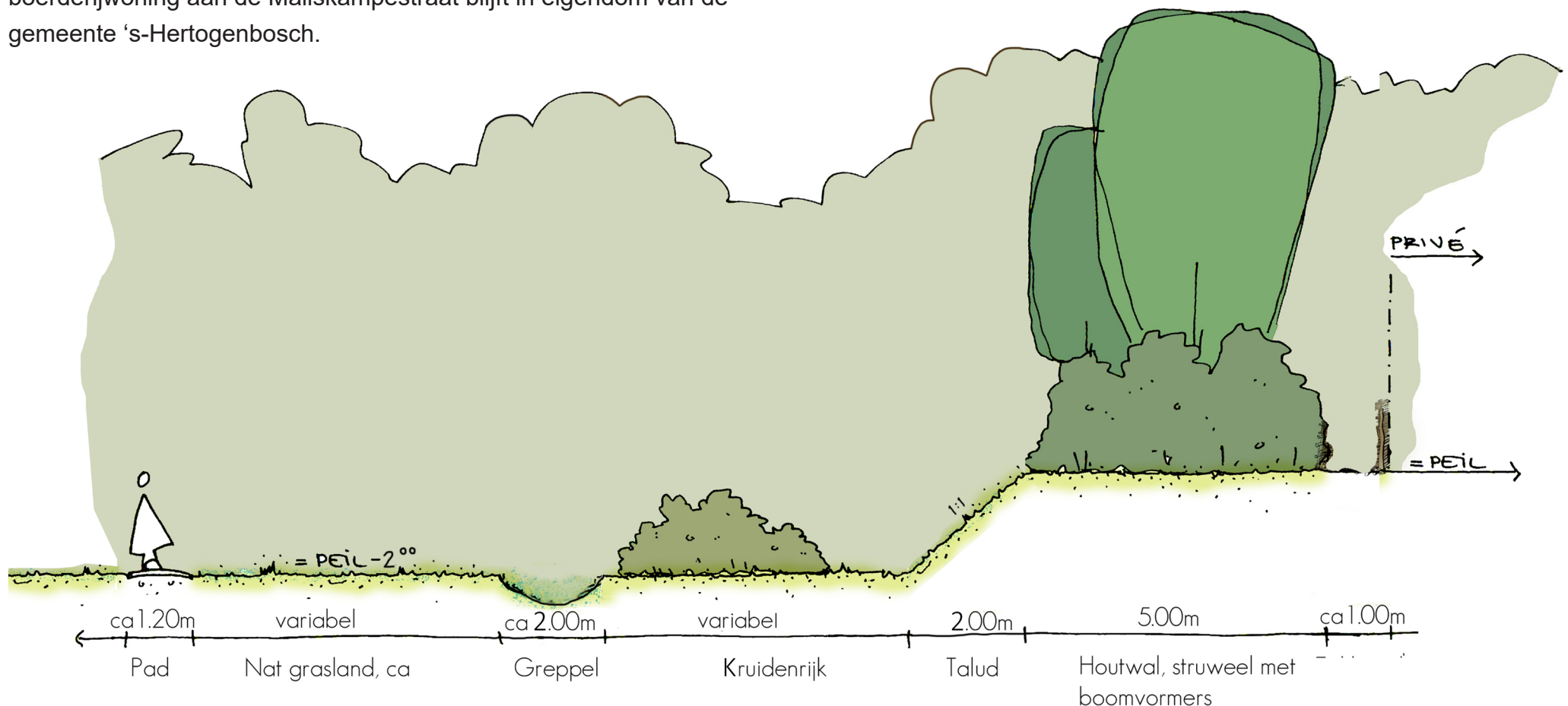
Dwarsprofiel: een houtwal markeert de grens tussen openbaar en privé
