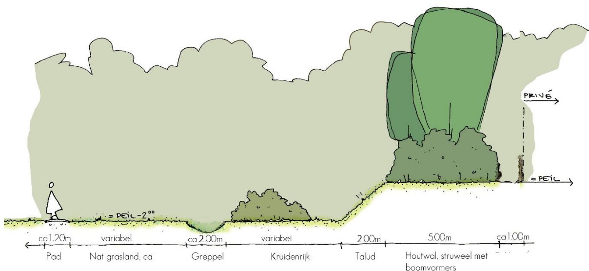
Figuur 3: Profiel houtwal
