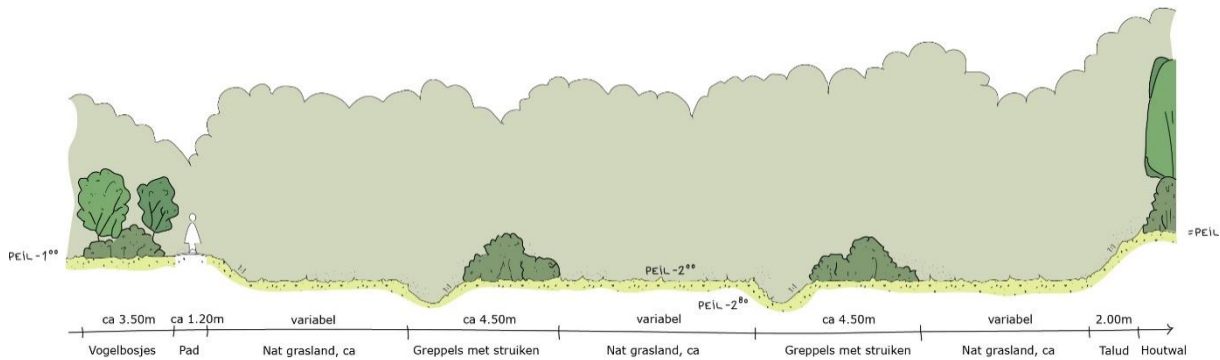
Figuur 5: profiel maaiveldverlaging met aan de rechterzijde de houtwal rondom de bouwkvelds en aan de linker zijde het voetpad met vogelbosjes.
