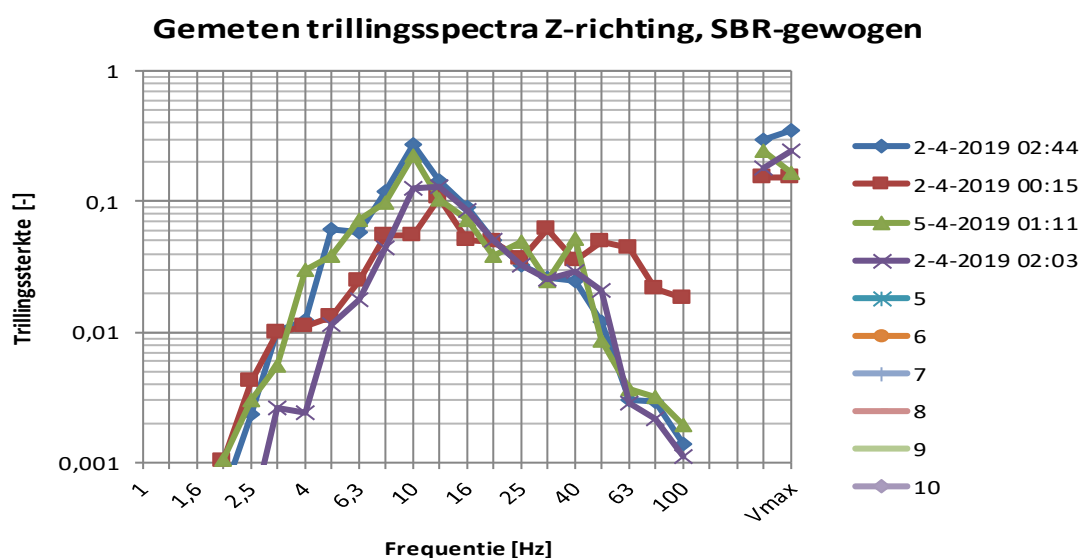
Figuur 5.1: Overzicht gewogen trillingspectra treinpassages meetpunt 1 gebruikt in prognose
