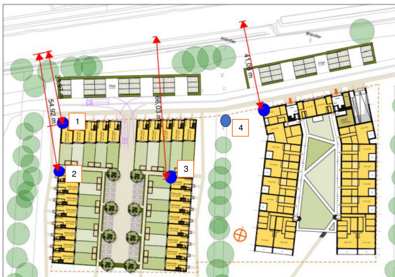
Figuur 3.1: Overzicht meetposities
