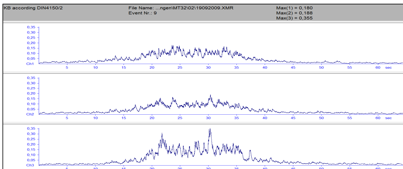
Figuur 4.1: Verloop voortschrijdende effectieve trillingssterkte maatgevende treinpassage meetpunt 1
