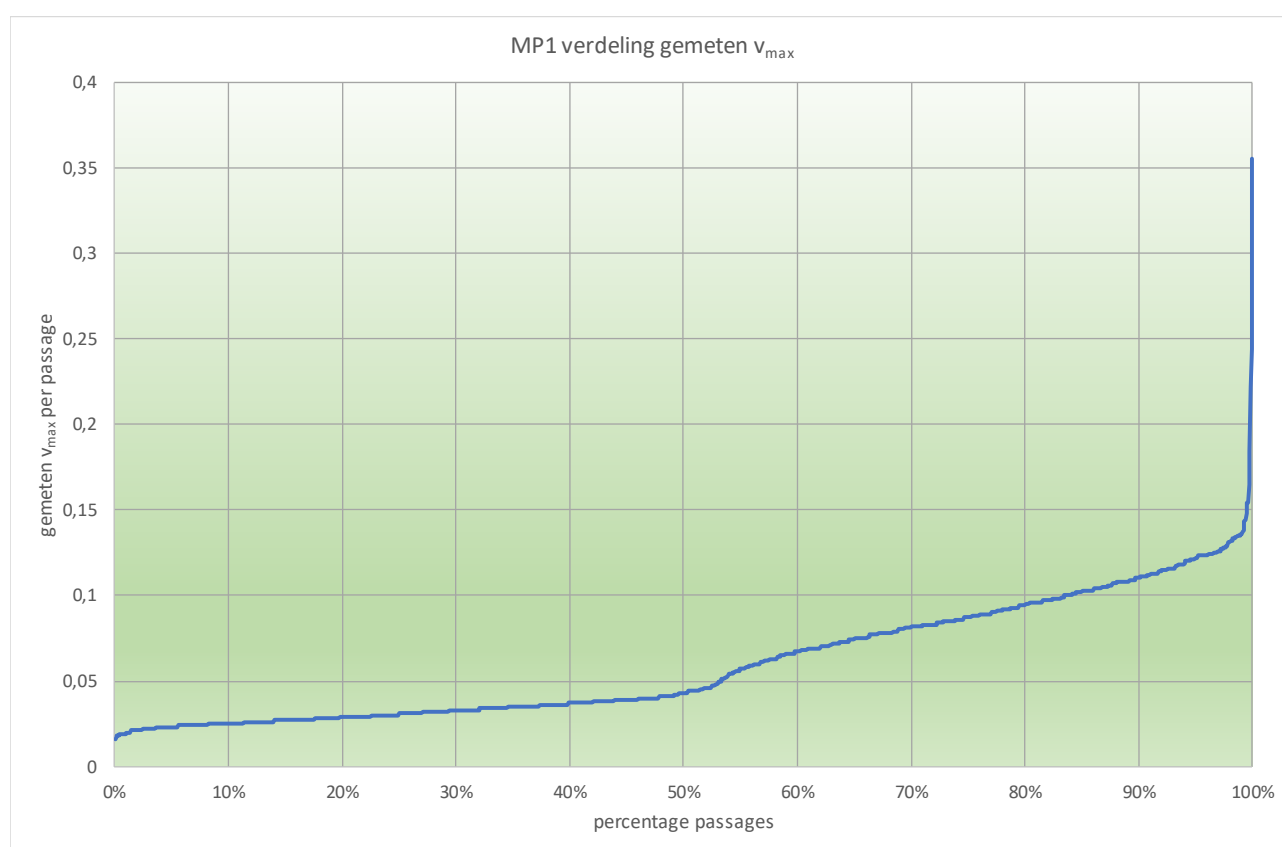
Figuur 5.4: Verdeling gemeten trillingssterkte op maaiveld meetpunt 1
