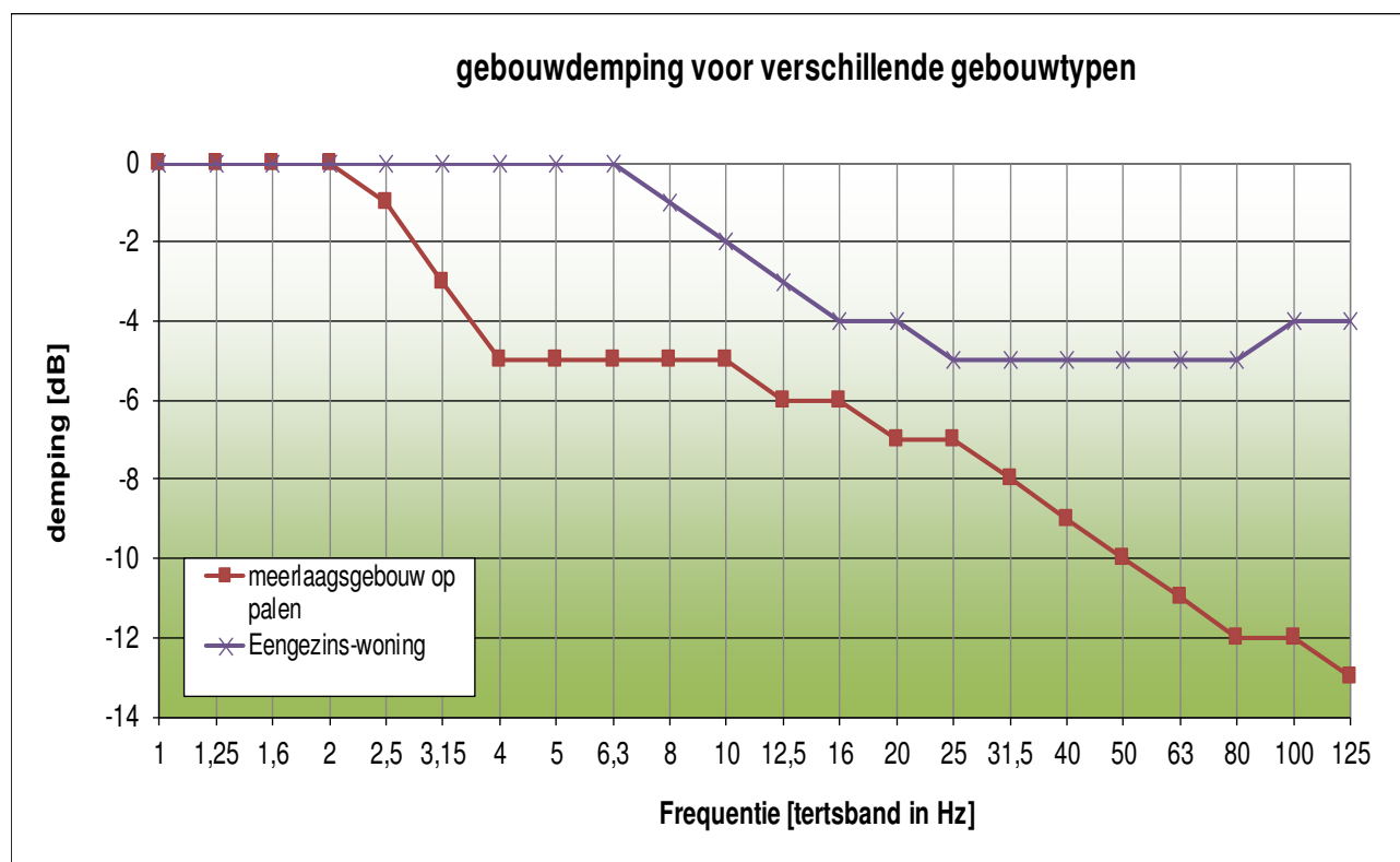
Figuur 5.2: Verloop overdrachtsfactor voor trillingen maaiveld naar fundering
