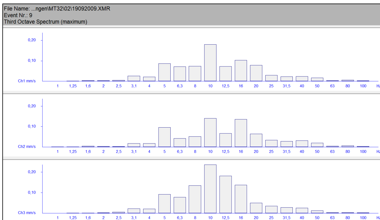
Figuur 4.2: Maxhold spectrum passage goederentrein figuur 4.1
