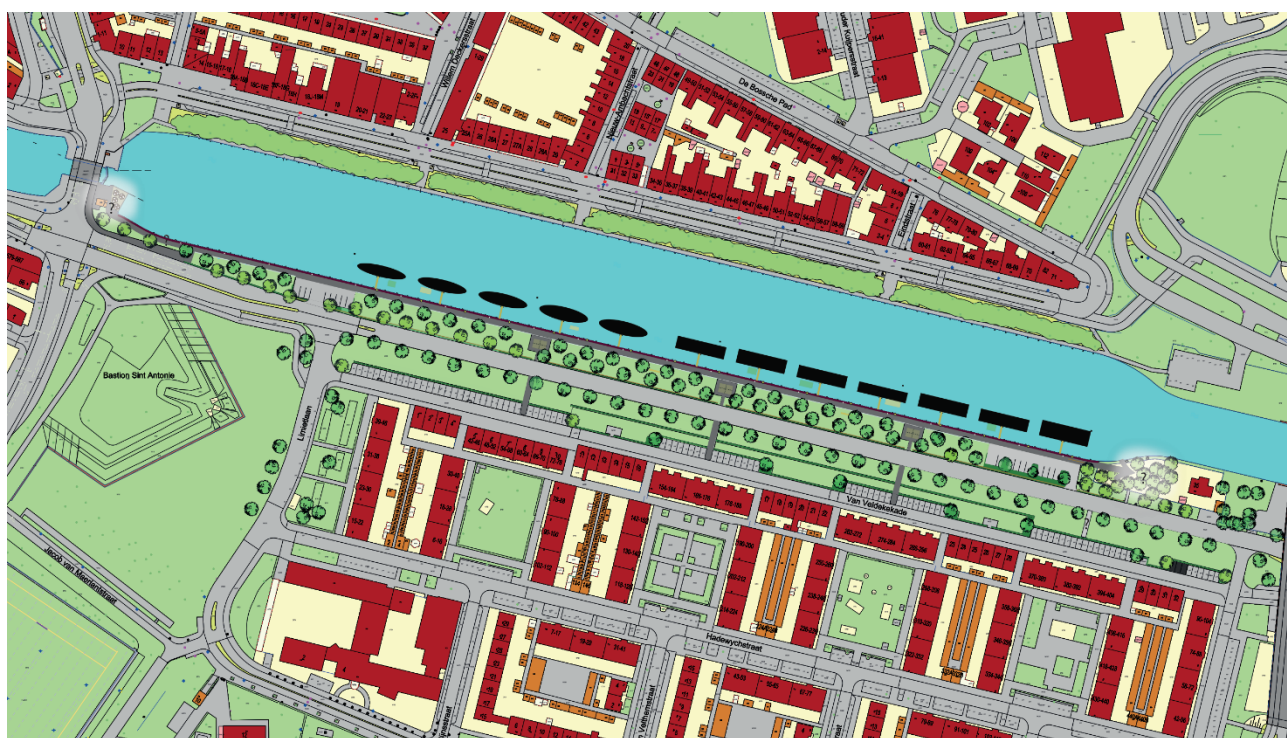
Figuur 3.1: Ontwerp woonbootligplaatsen Van Veldekekade
