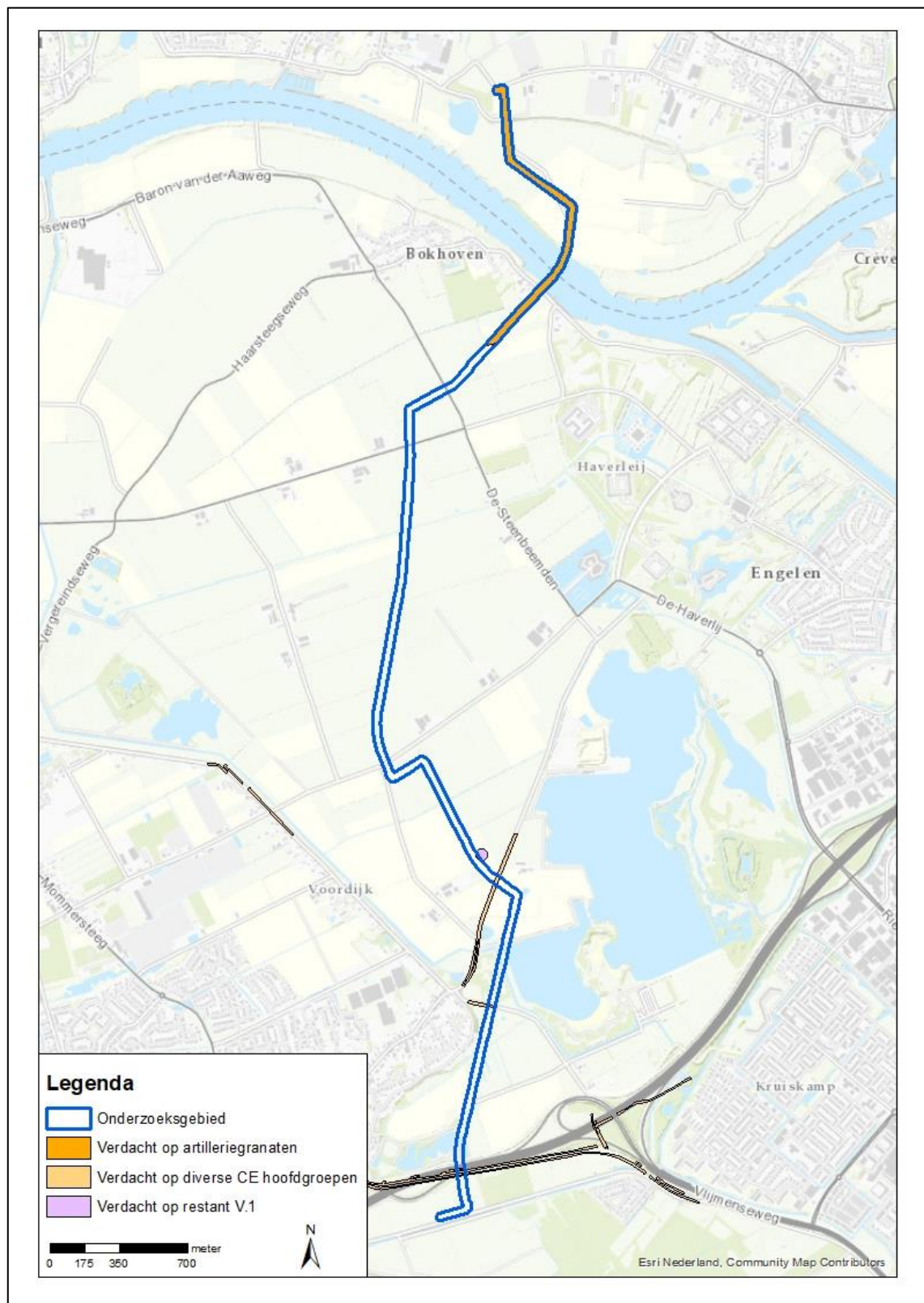
Afbeelding 14: CE-bodembelastingkaart onderzoeksgebied.
