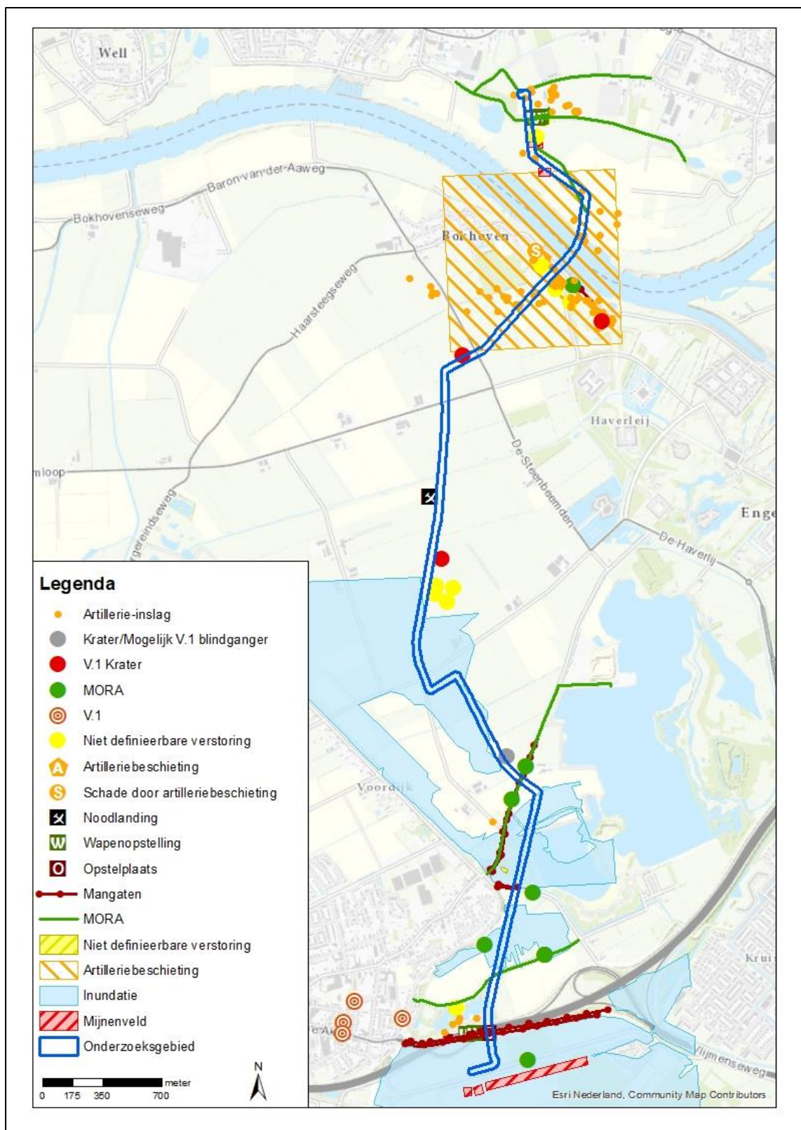
Afbeelding 12: Inventarisatiekaart onderzoeksgebied.
