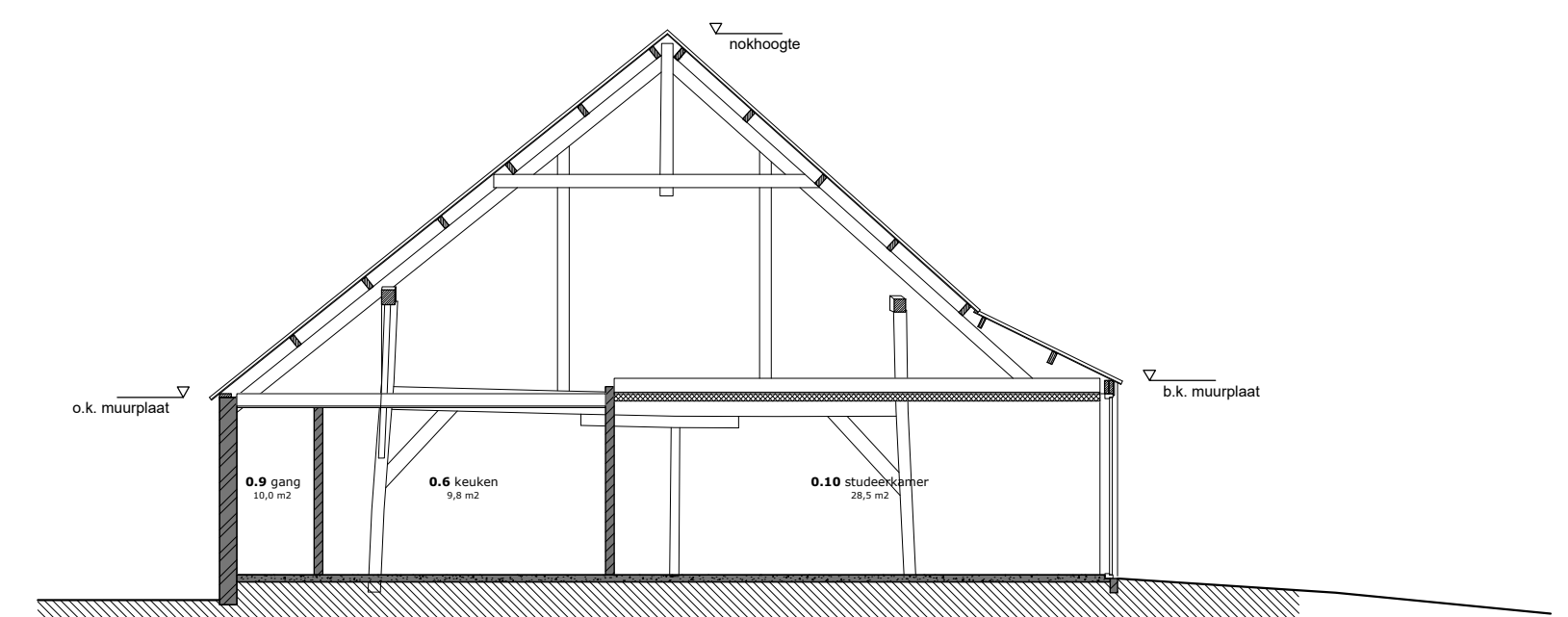
Doorsnede C-C
