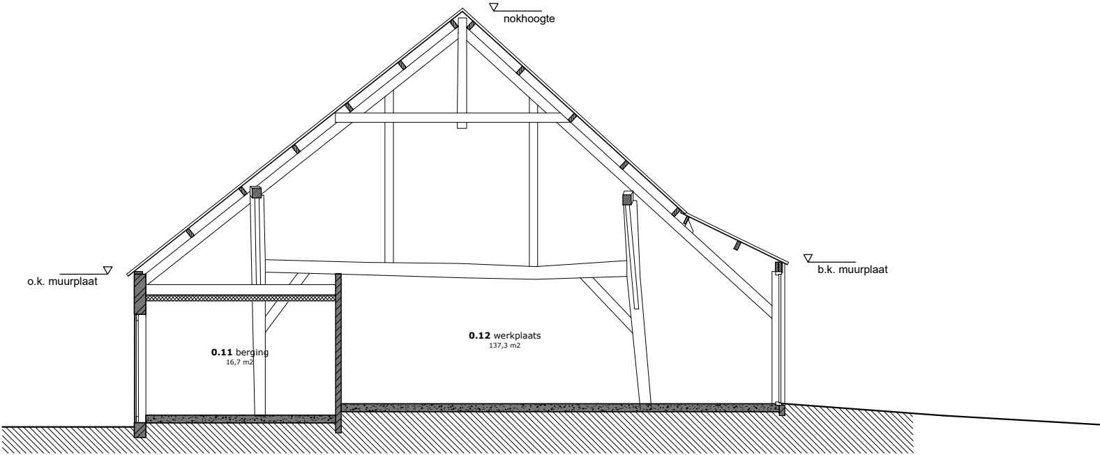
Doorsnede D-D
