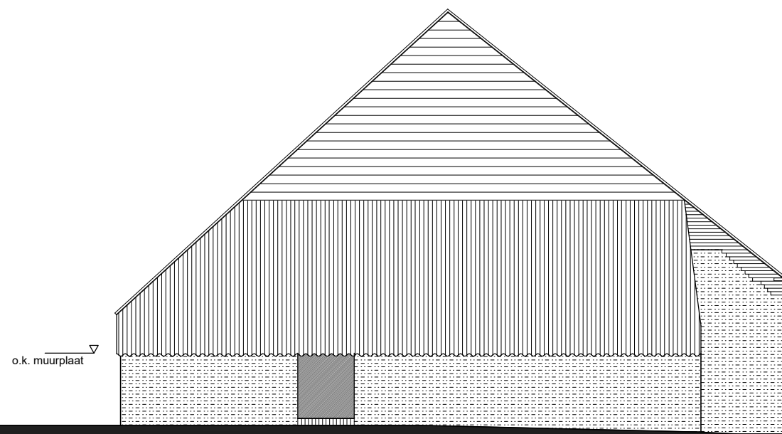
achtergevel west-georiënteerd
