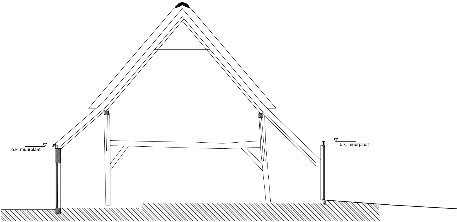
Doorsnede D-D
