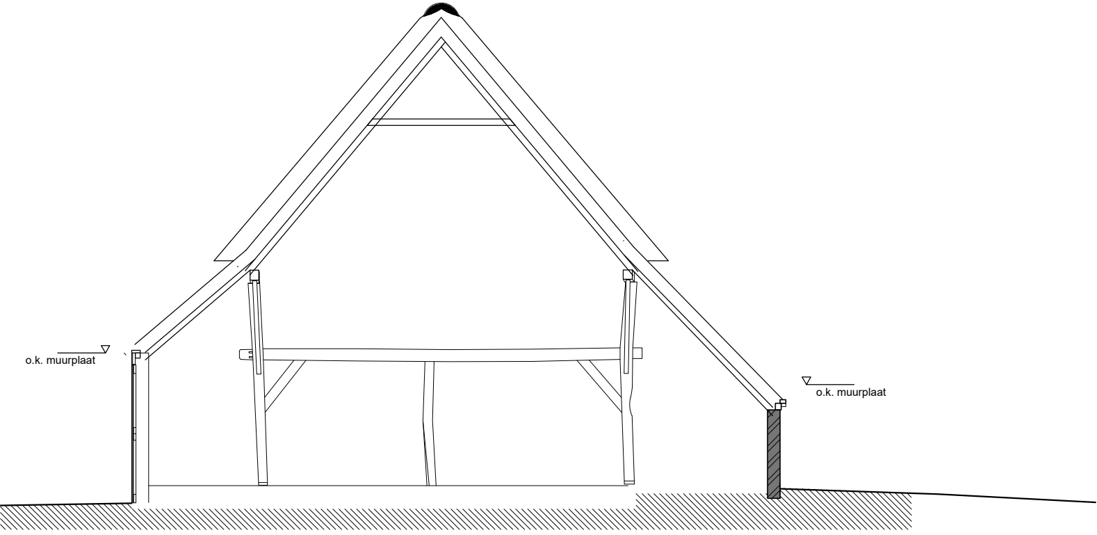
Doorsnede E-E
