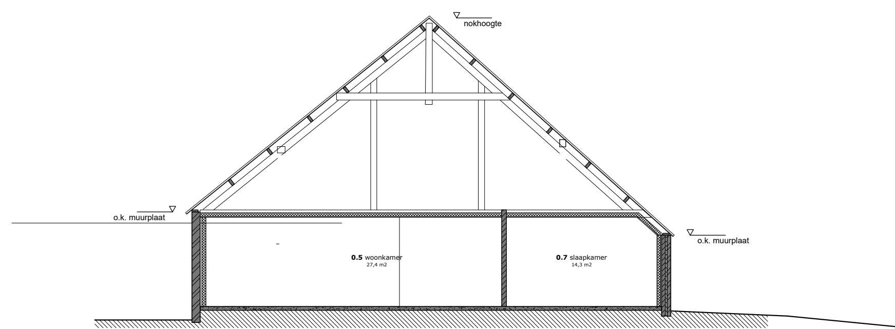
Doorsnede A-A
