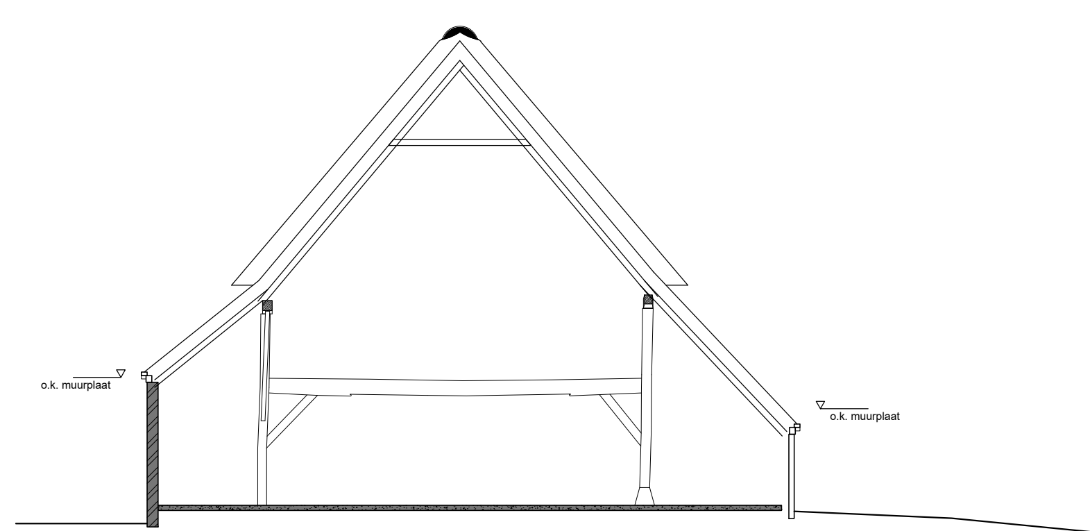
Doorsnede B-B
