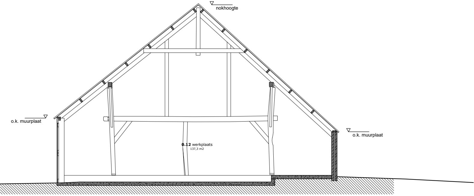
Doorsnede E-E
