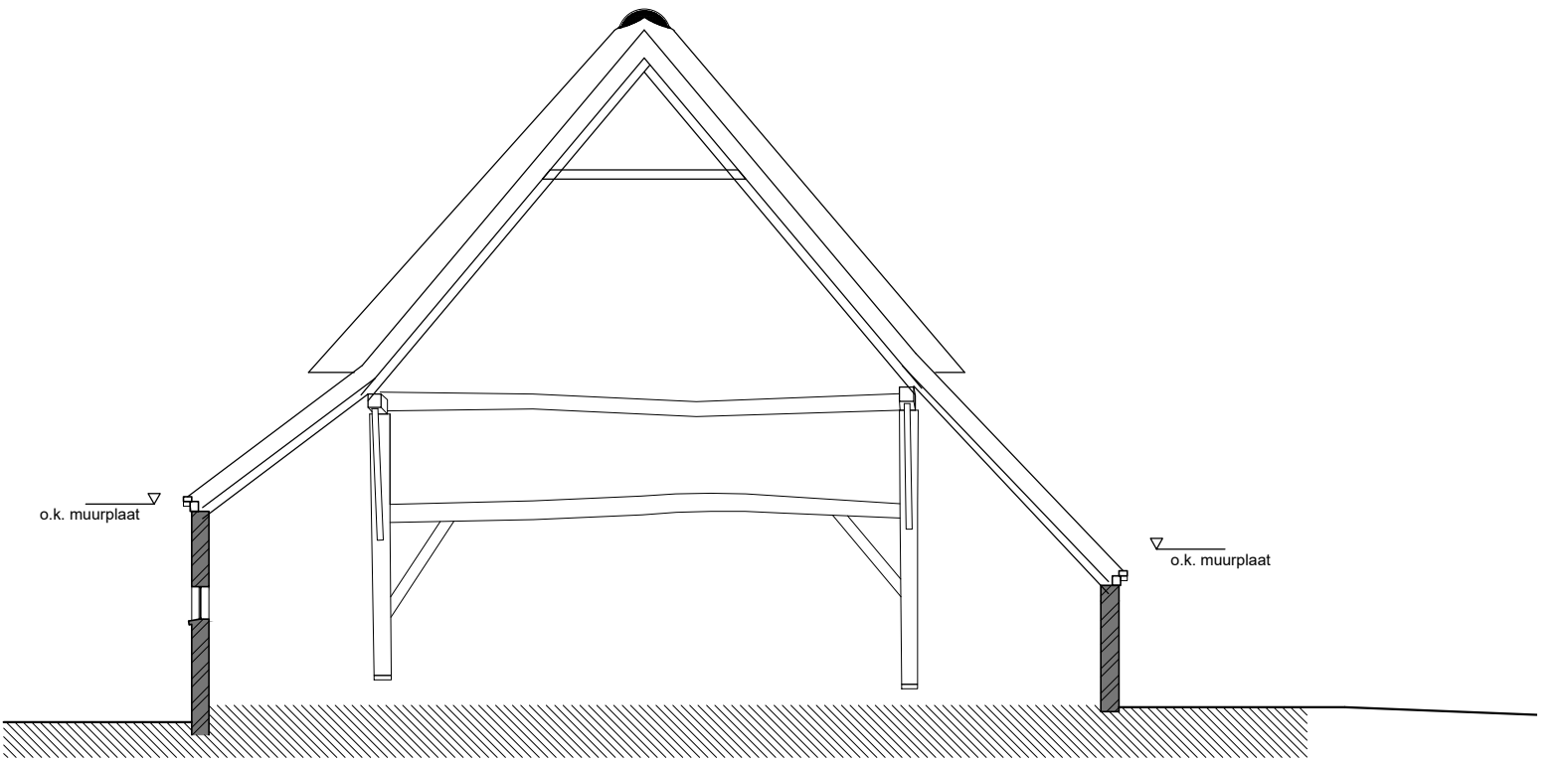
Doorsnede F-F
