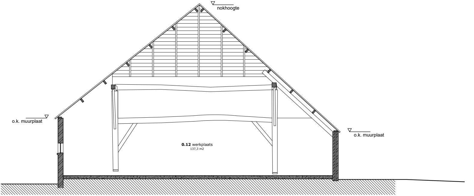
Doorsnede F-F
