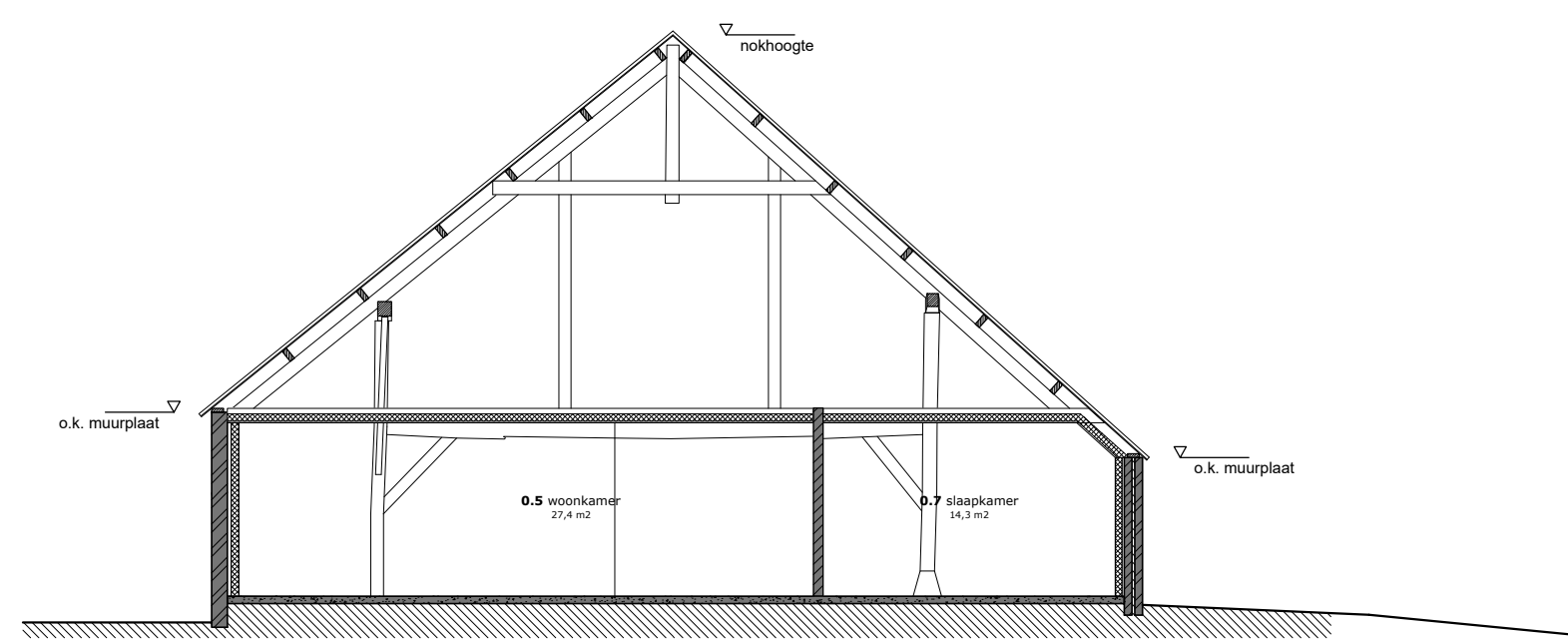
Doorsnede B-B
