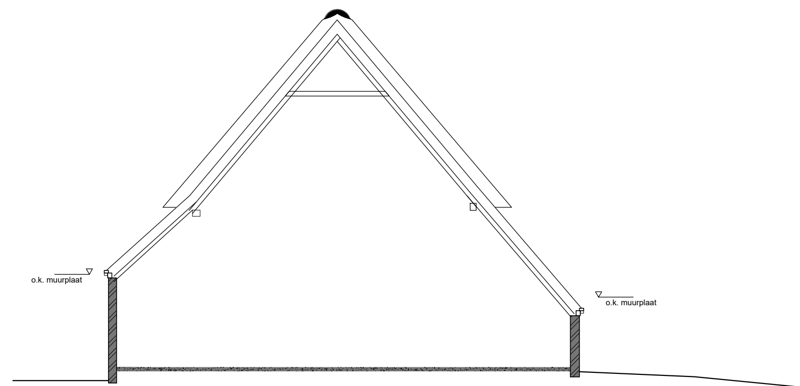
Doorsnede A-A
