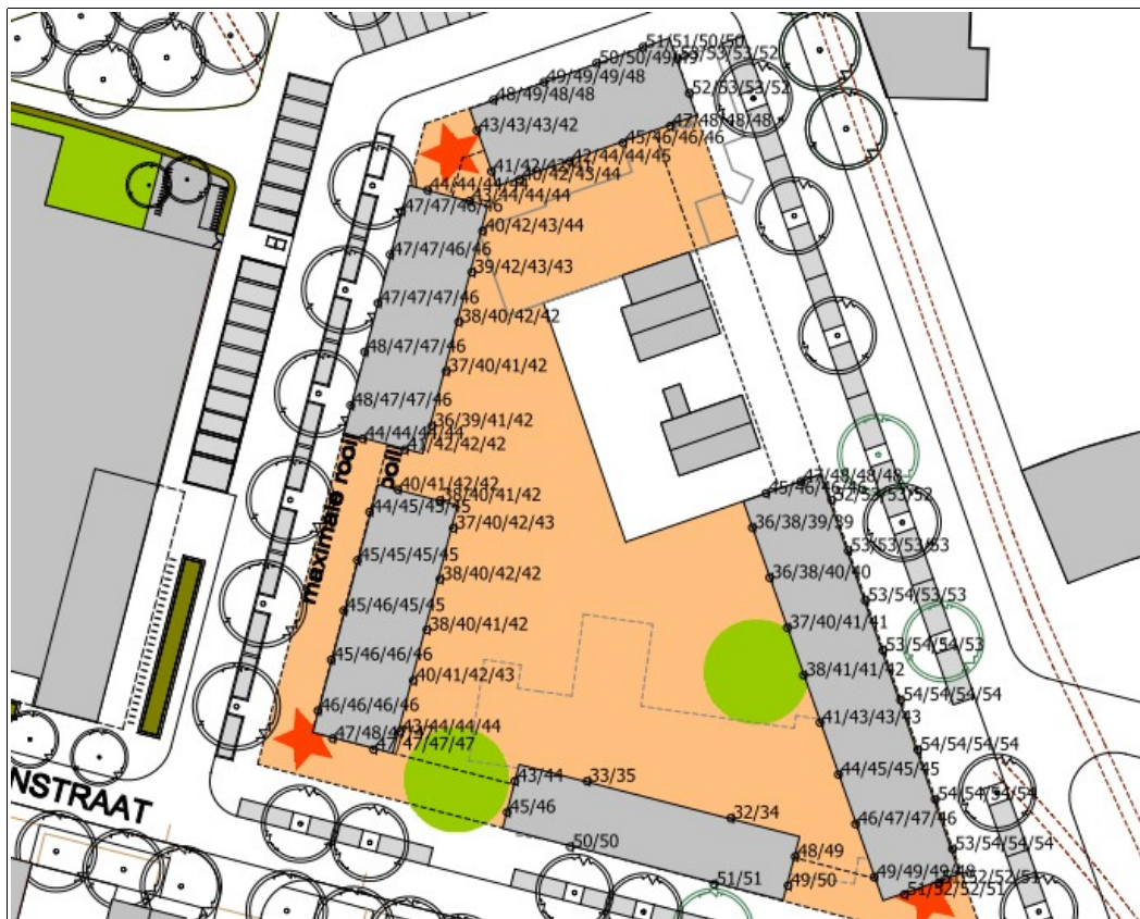
f4.1 Geluidbelastingen L_{den} in dB vanwege wegverkeer (alle wegen gecumuleerd), incl. aftrek art. 110g Wgh, planvariant B1
