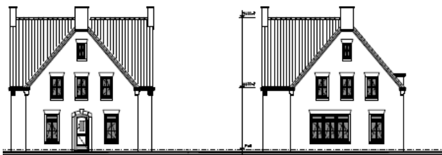
Aanzicht voorgevel en rechter zijgevel (Bron: Arceau Architecten, 2011)
