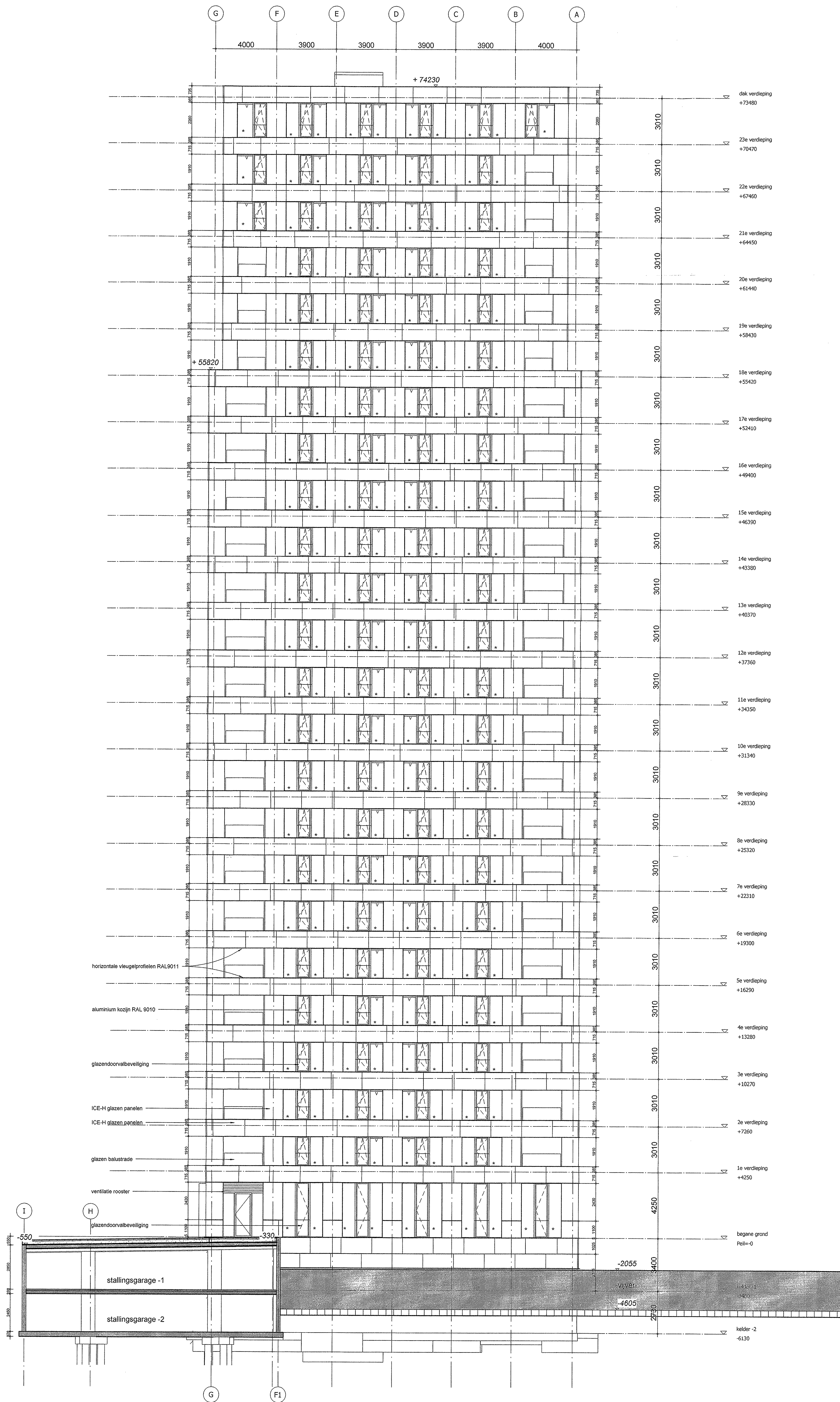
Noordgevel
