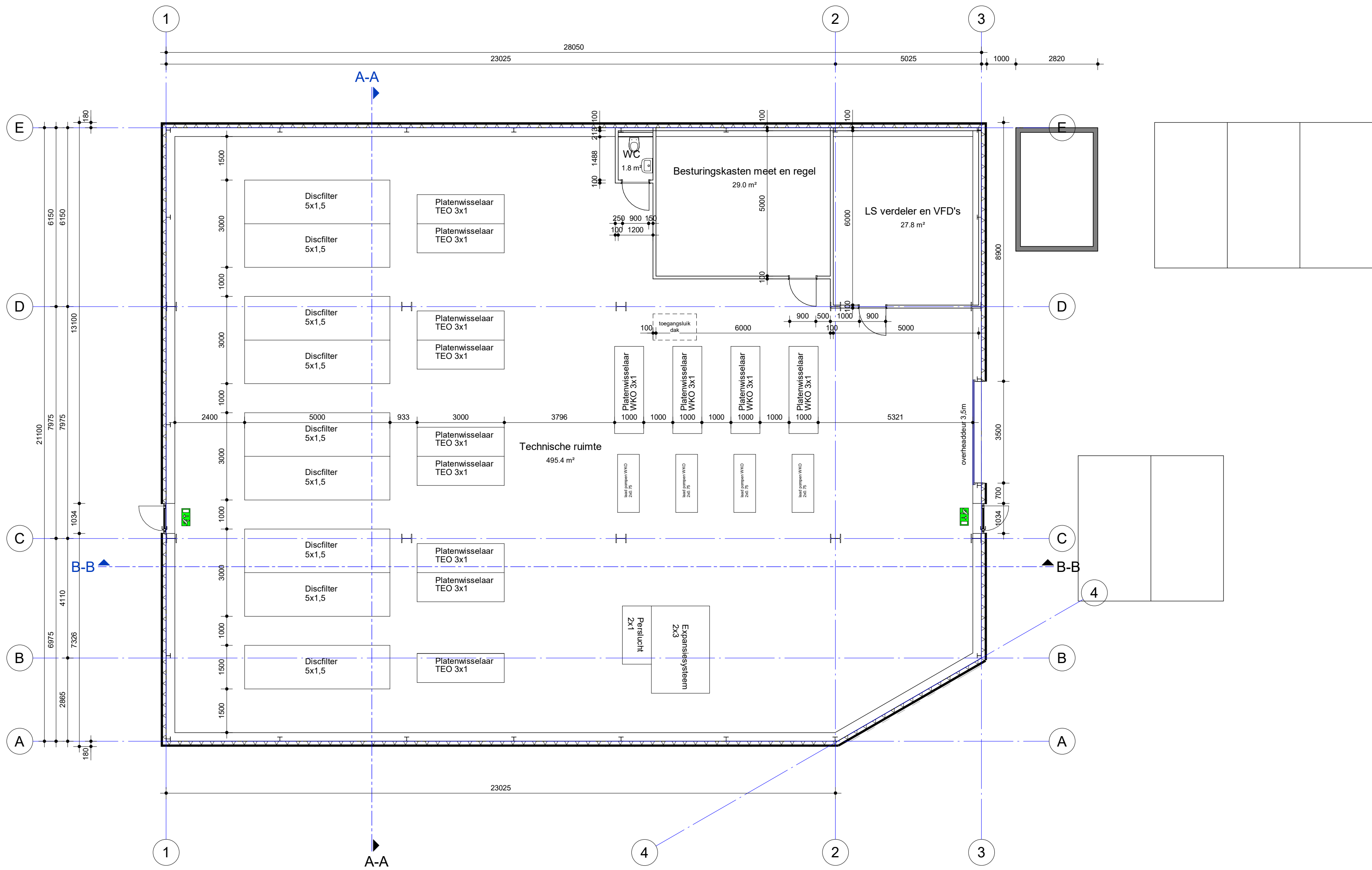
begane grond (schaal 1 : 100)
