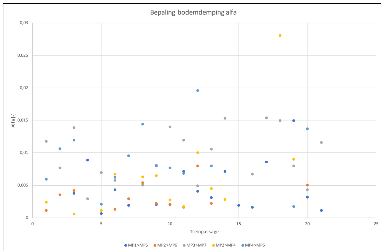
Figuur 5.4: Berekende bodemdemping alfa
