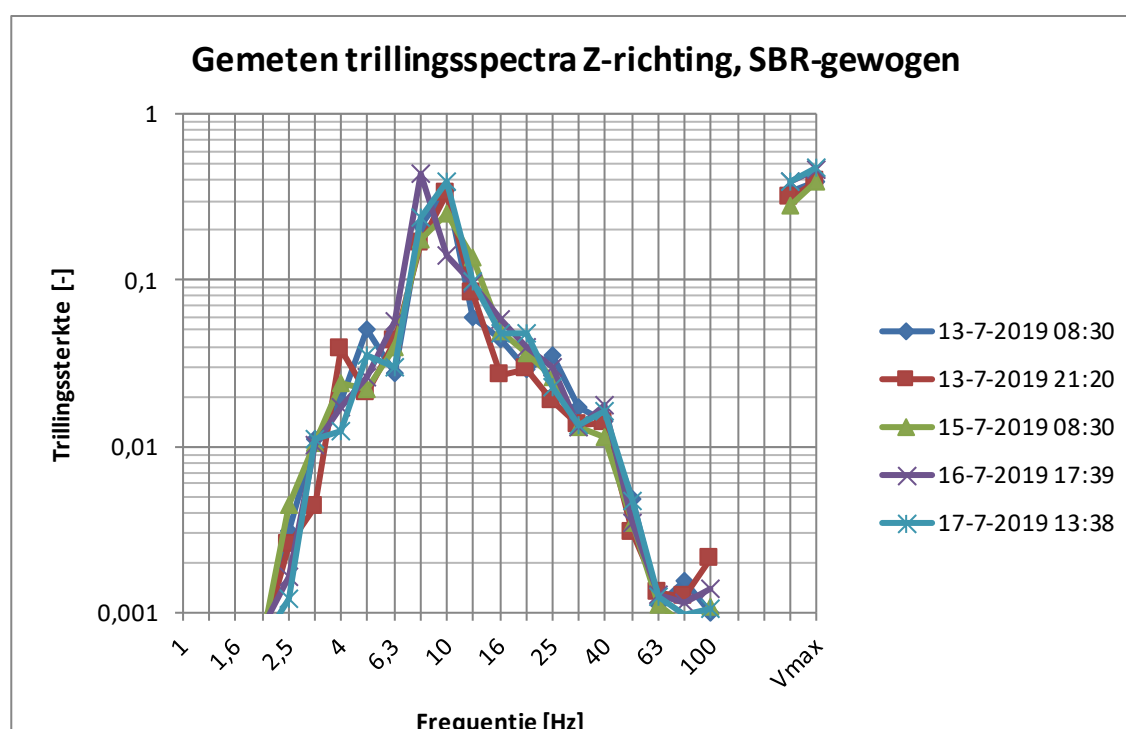
Figuur 5.1: Overzicht gewogen trillingsspectra treinpassages meetpunt 3 in prognose
