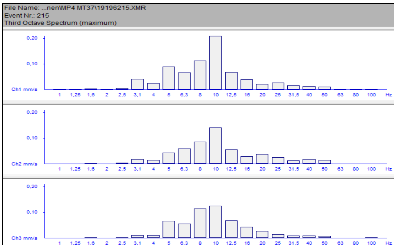
Figuur 4.3: Max hold frequentiespectrum passage 15 juli om 18.52 uur van meetpunt 4
