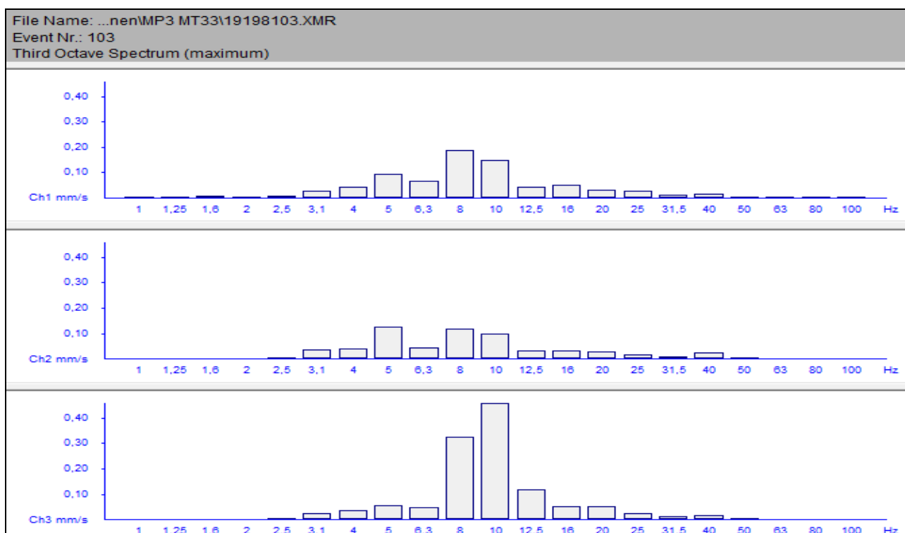
Figuur 4.2: Maxhold spectrum passage goederentrein figuur 4.1
