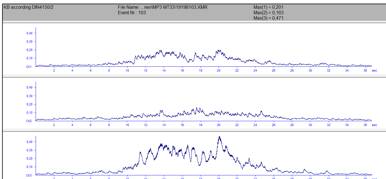
Figuur 4.1: Verloop voortschrijdende effectieve trillingssterkte treinpassage met hoogste V_{\max} (MP3)
