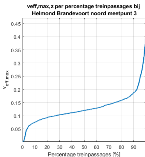
Figuur 5.5: Cumulatieve verdeling v_{\text{max}} per treinpassage voor meetpunt 3
