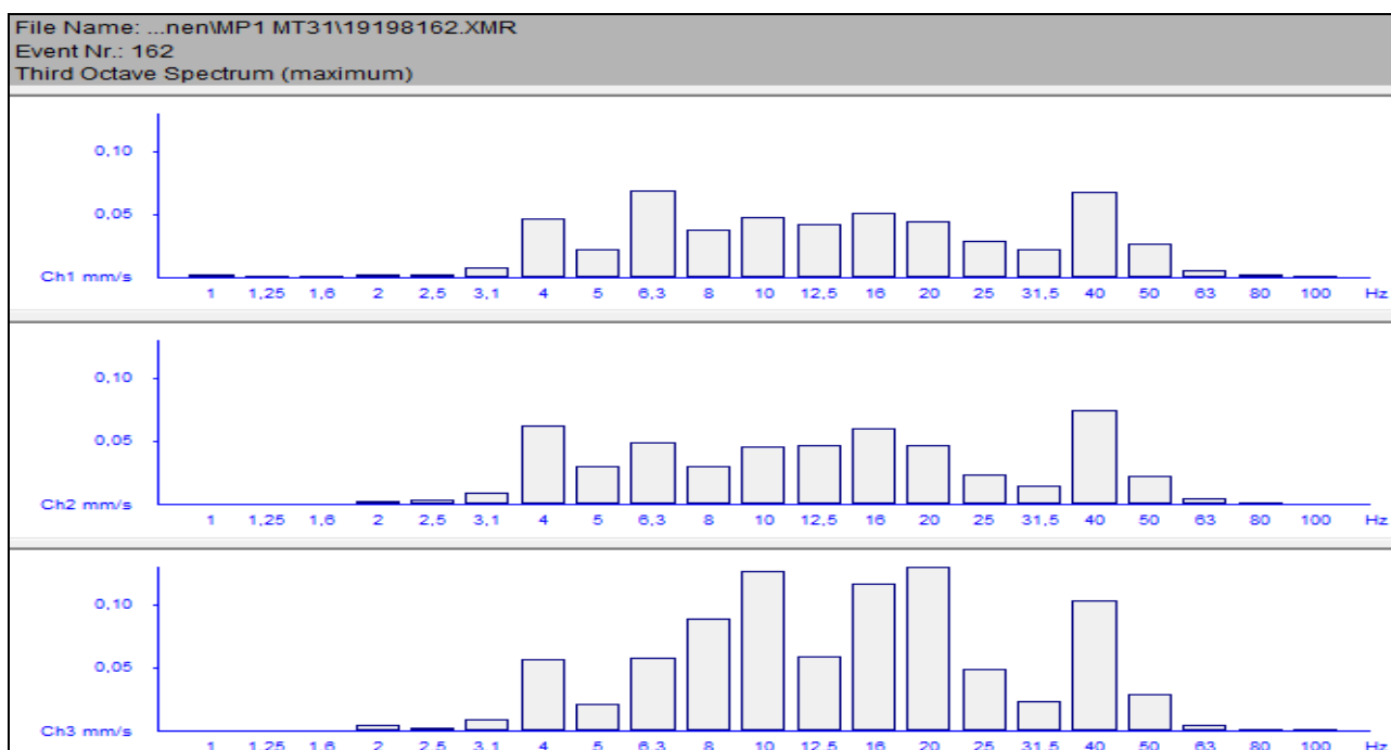
Figuur 4.4: Max hold frequentiespectrum passage 17 juli om 20.08 uur van meetpunt 1
