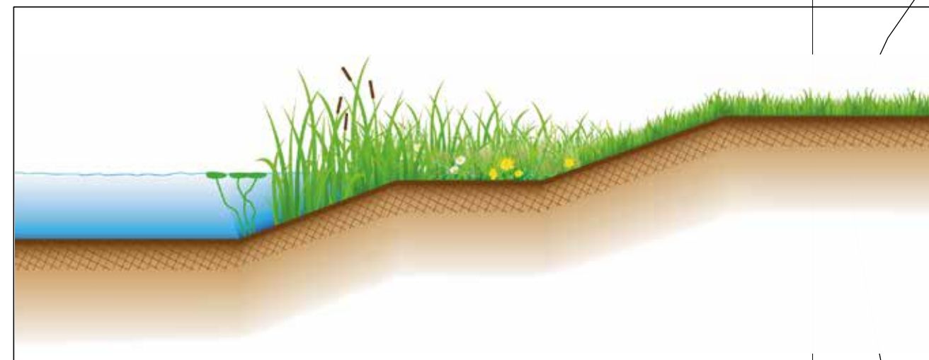
Profiel ecologische oever
