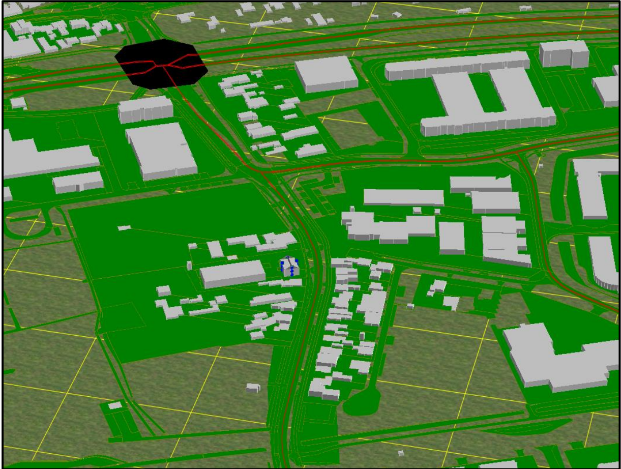
Afbeelding 4. Rekenmodel, 3d-weergave
