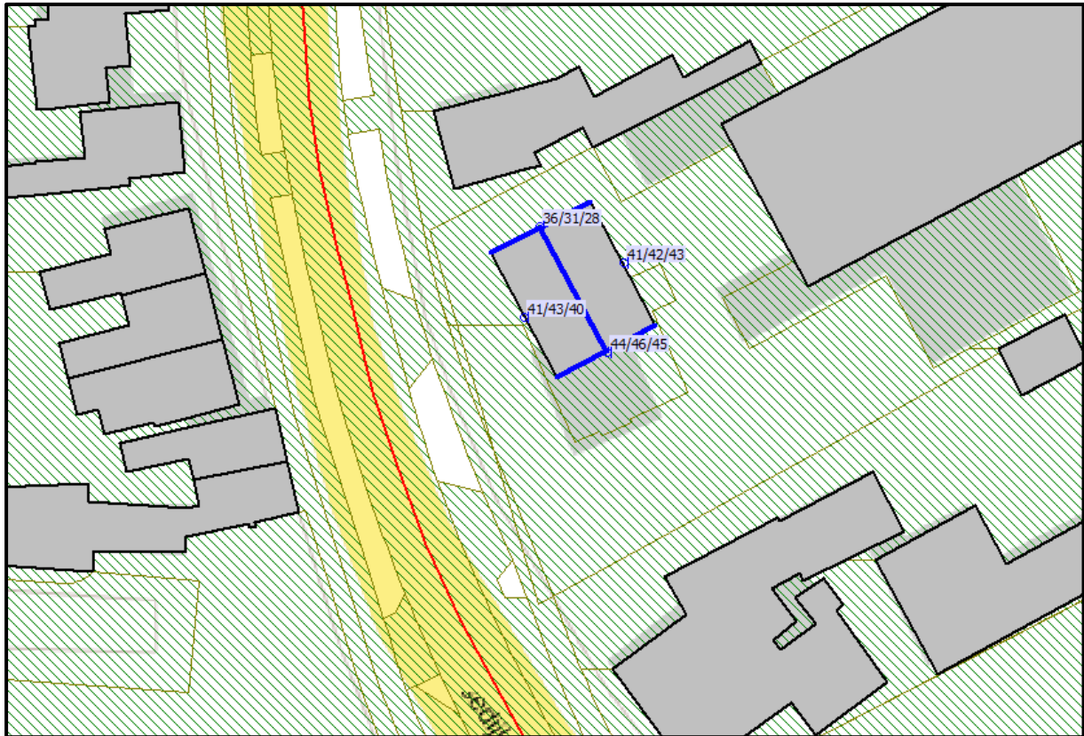
Afbeelding 6. Geluidbelastingen L_{den} (incl. aftrek art. 110g Wgh) Europaweg
