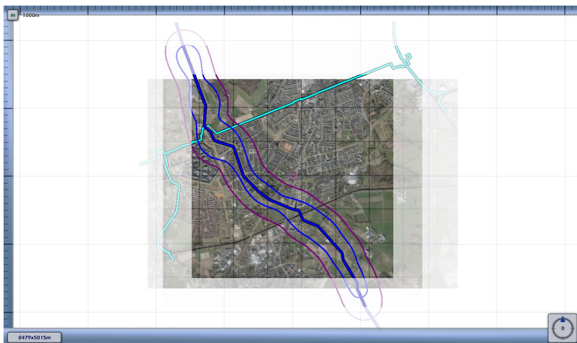
3.2 Figuur 3.2 Plaatsgebonden risico voor 9058_leiding-Z-514-01-deel-1 van N.V. Nederlandse Gasunie
