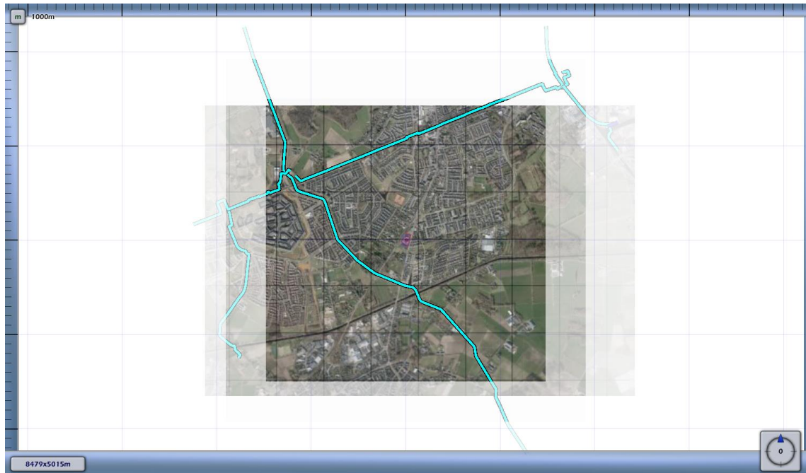
3.12 Figuur 3.12 Plaatsgebonden risico voor 9058_leiding-Z-540-44-deel-1 van N.V. Nederlandse Gasunie
