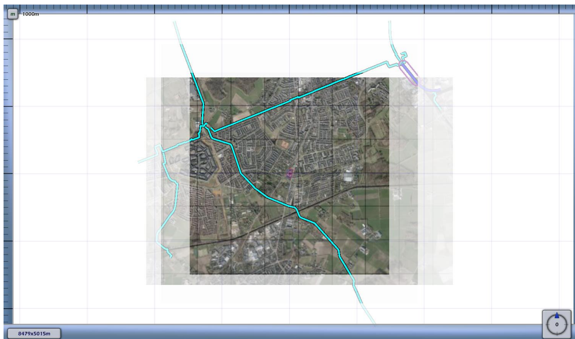
3.10 Figuur 3.10 Plaatsgebonden risico voor 9058_leiding-Z-540-01-deel-2 van N.V. Nederlandse Gasunie
