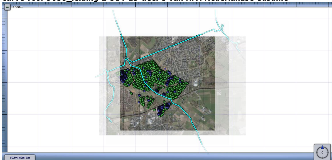
Figuur 4.7 Kilometer leiding behorende bij de maximale overschrijding van de FN-curve voor 9058_leiding-Z-514-15-deel-3 van N.V. Nederlandse Gasunie
