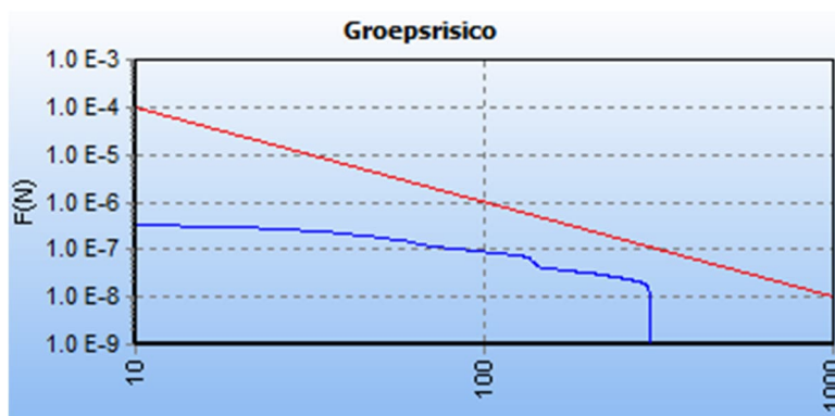
Afbeelding 7 fN-curve buisleiding A-521-deel-1, beoogde situatie
