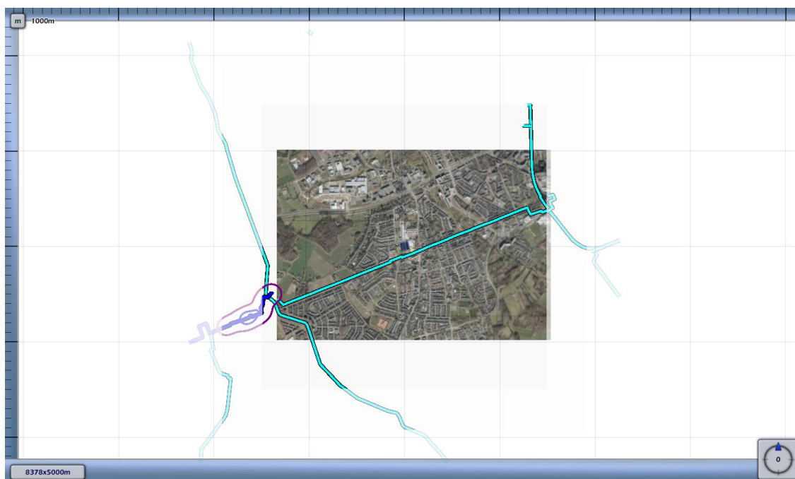
3.4 Figuur 3.4 Plaatsgebonden risico voor 7872_leiding-Z-514-06-deel-1 van N.V. Nederlandse Gasunie
