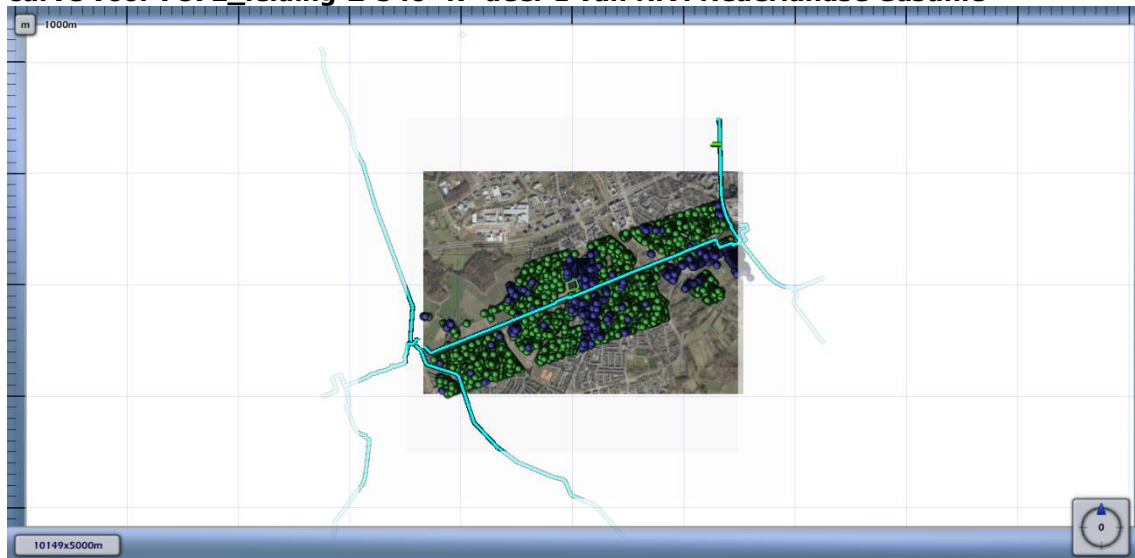
Figuur 4.9 Kilometer leiding behorende bij de maximale overschrijding van de FN-curve voor 7872_leiding-Z-540-47-deel-1 van N.V. Nederlandse Gasunie
