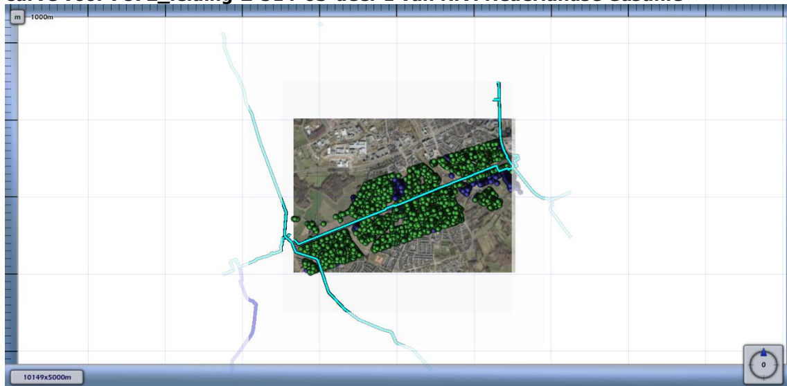
Figuur 4.3 Kilometer leiding behorende bij de maximale overschrijding van de FN-curve voor 7872_leiding-Z-514-03-deel-1 van N.V. Nederlandse Gasunie
