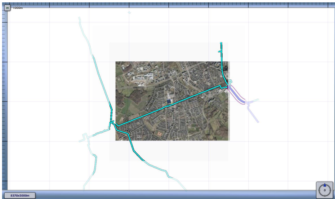
3.6 Figuur 3.6 Plaatsgebonden risico voor 7872_leiding-Z-540-01-deel-1 van N.V. Nederlandse Gasunie
