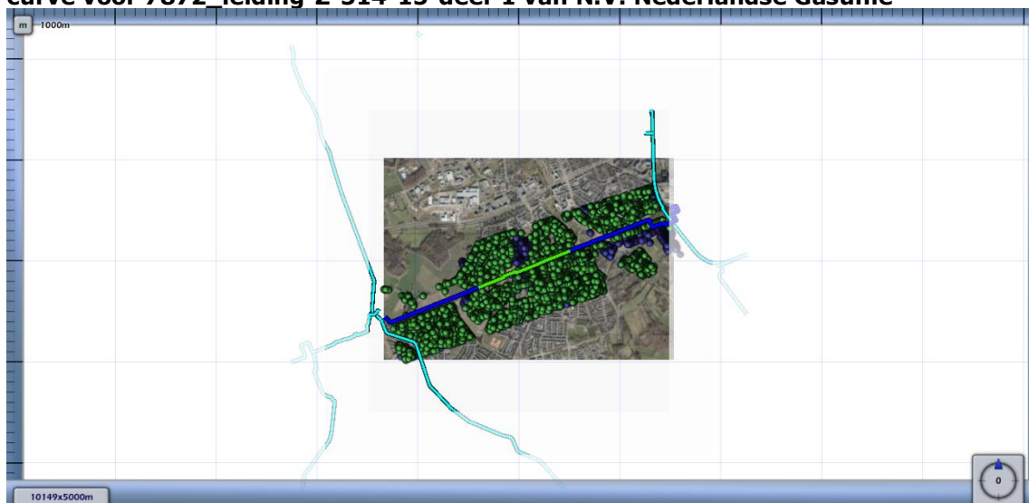
Figuur 4.5 Kilometer leiding behorende bij de maximale overschrijding van de FN-curve voor 7872_leiding-Z-514-15-deel-1 van N.V. Nederlandse Gasunie
