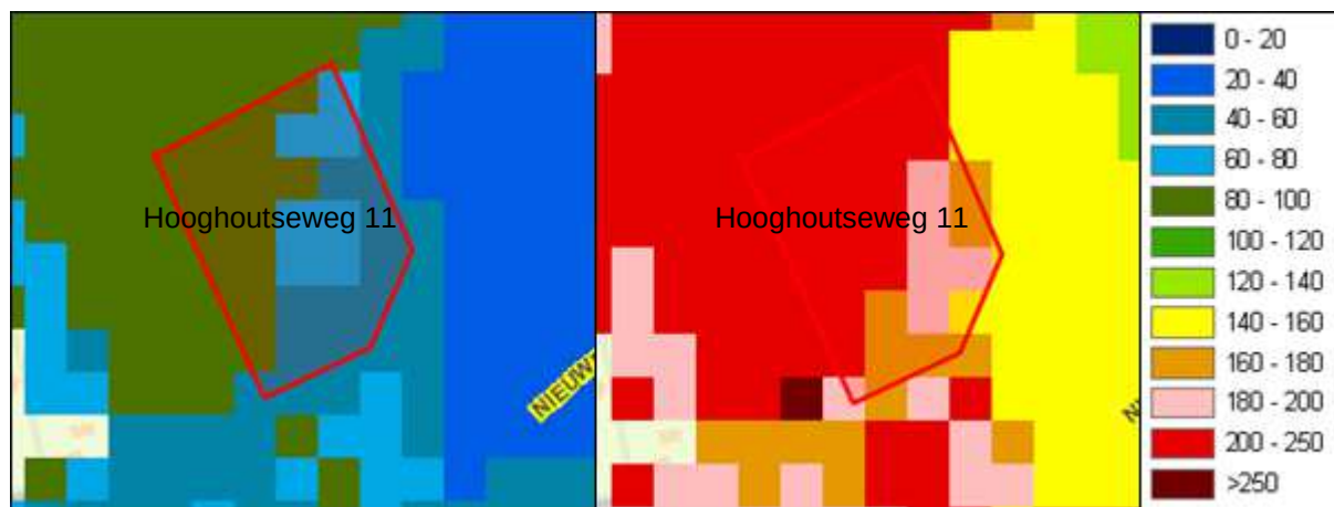
Figuur 16: GHG en GLG ter plaatse van het plangebied
