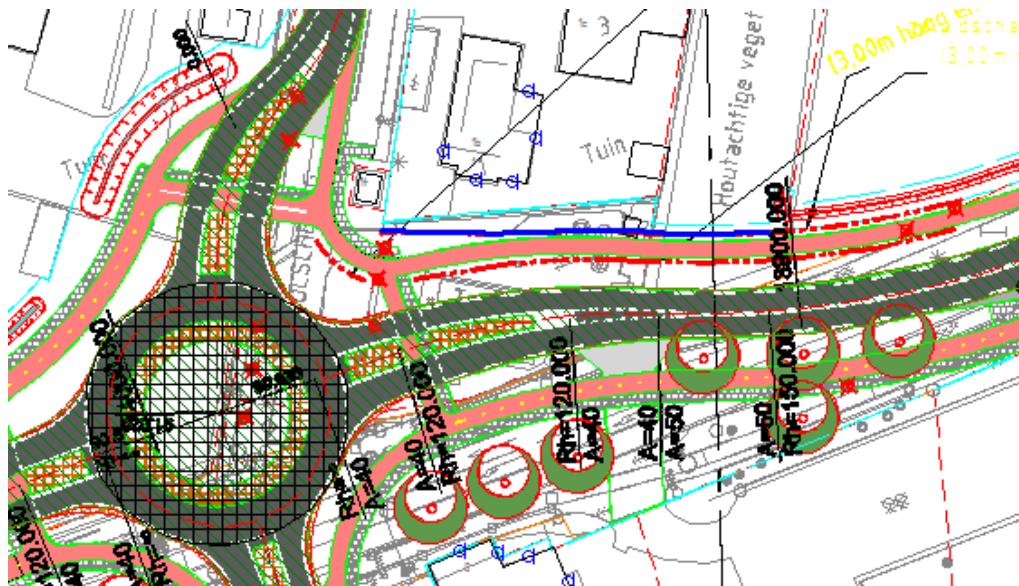
Figuur 20: Situering scherm Tolschestraat
