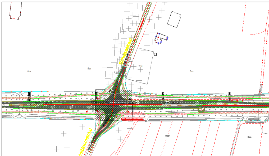
Figuur 6: Toekomstige situatie kruising N324-Scheisestraat
