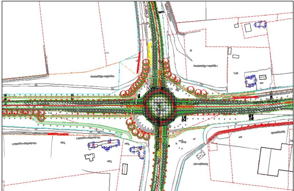
Figuur 8: Toekomstige situatie kruising N324-N277
