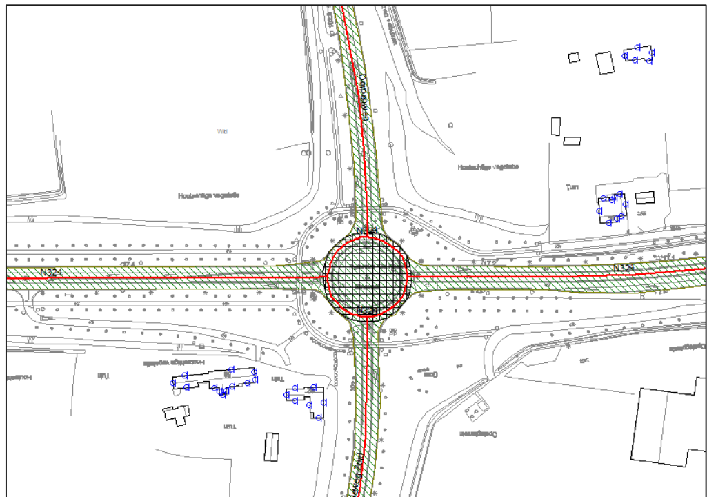
Figuur 7: Huidige situatie kruising N324-N277
