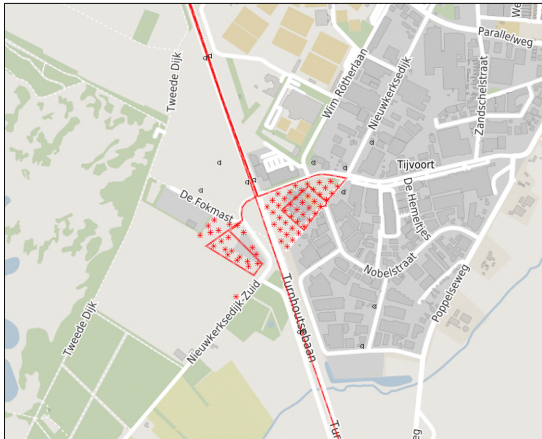
Figuur 3.2: Overzicht rijlijnen en emissiebronnen op het terrein van de inrichting
