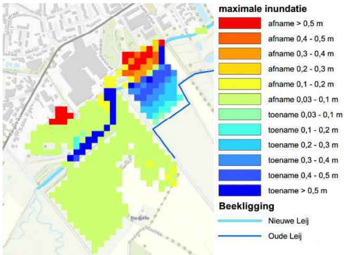
Figuur 5-4: verschil in inundatie bij een hydrologische situatie T=10
