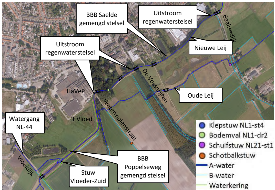
Figuur 2-8: Ligging Nieuwe en Oude Leij [bron: Beheerregister Waterschap De Dommel]
