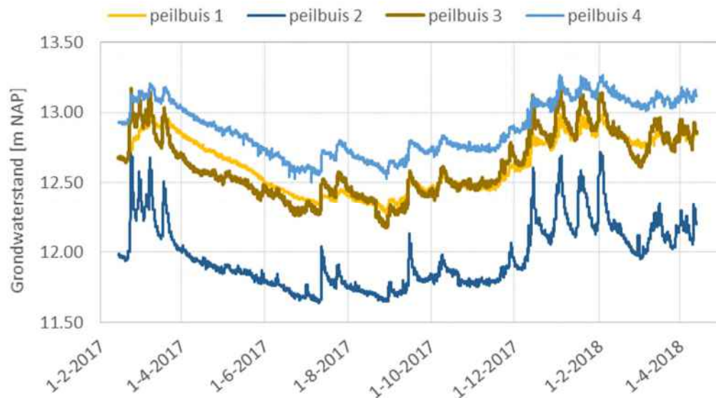
Figuur 2-7: Waarnemingen lokale peilbuizen Zuidrand Goirle
