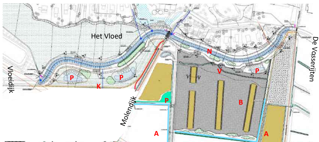
Figuur 4-1: Indicatief beeld van het Definitief Ontwerp van de groenblauwe zone
