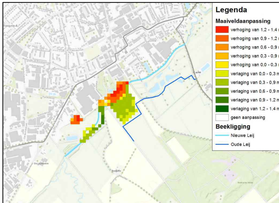
Figuur 4-6: Verhoging (rood) of verlaging (groen) maaiveld in m, verschil huidige situatie en Definitief Ontwerp
