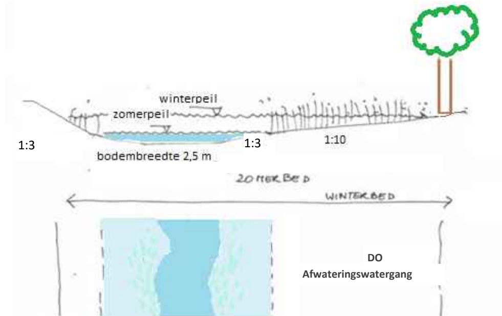
Figuur 4-2: Principeprofiel Nieuwe Leij
