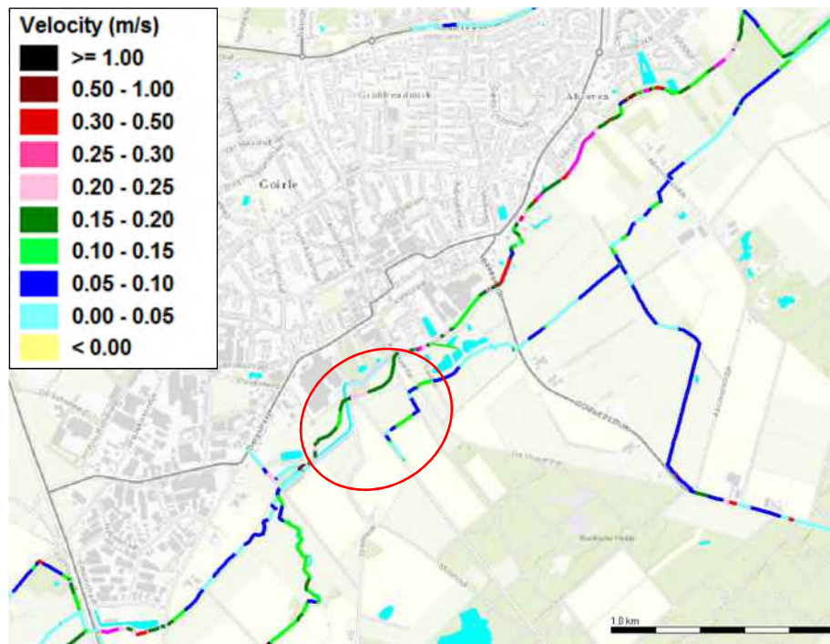
Figuur 5-1: Stroomsnelheid in m/s bij zomerafvoer, definitief ontwerp, rode cirkel is plangebied
