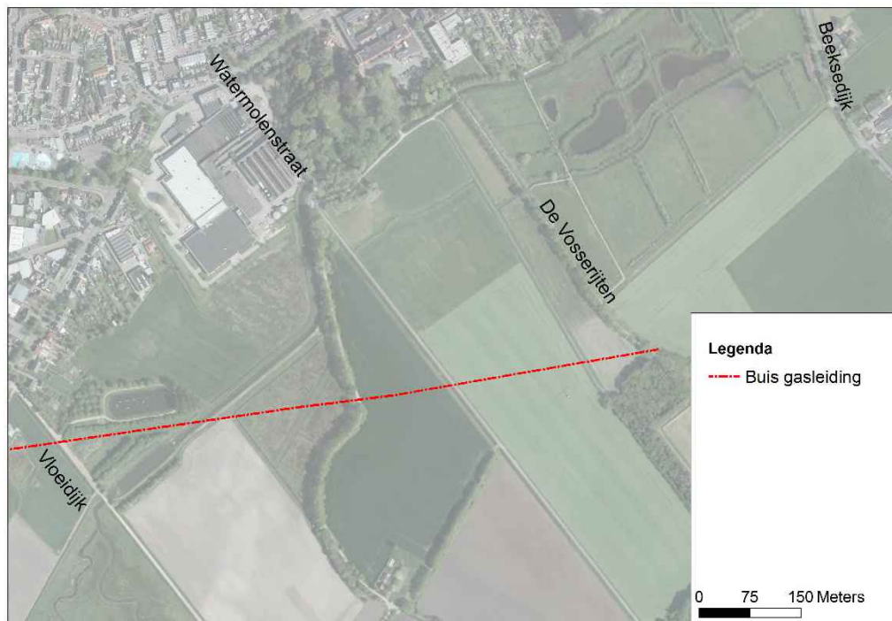
Figuur 2-12: Indicatieve ligging van de gasleiding [Bron: Ruimtelijke plannen.nl]
