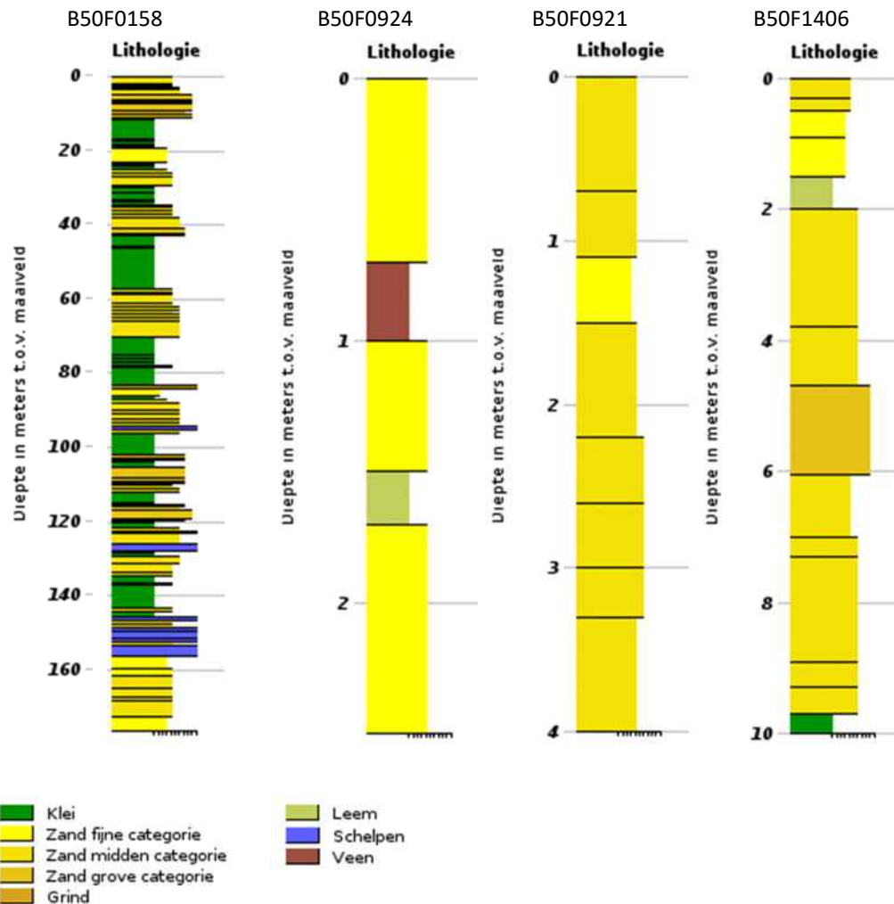
Figuur 2-3: Boorprofielen in de omgeving van het plangebied [bron: Dinoloket, TNO]
