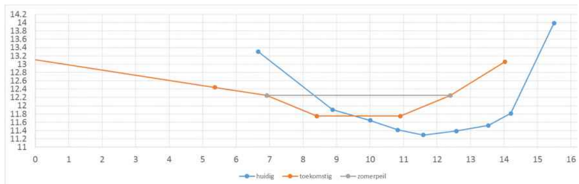
Figuur 4-3: Vergelijking profiel huidige (blauw) en toekomstige situatie (oranje) ter hoogte van het Vloed.
