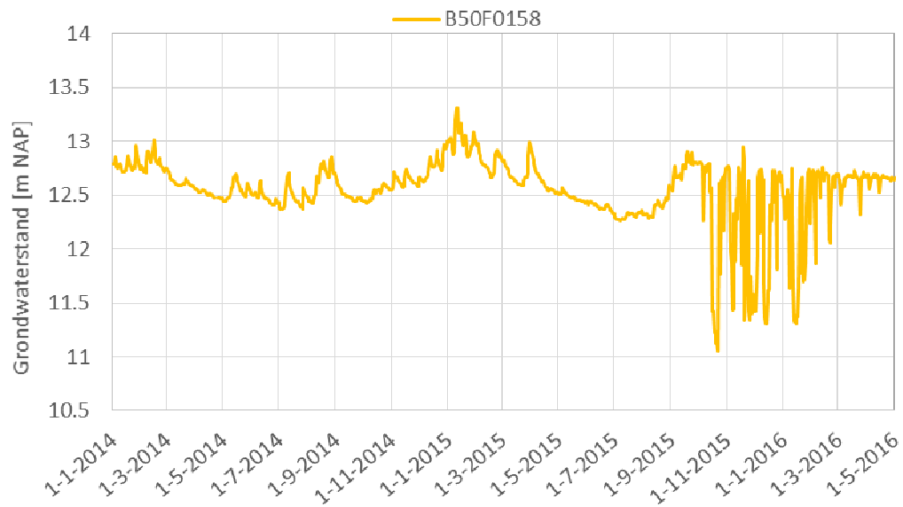
Figuur 2-5: Peilbuis B50F0158 [bron: Dinoloket, TNO]
