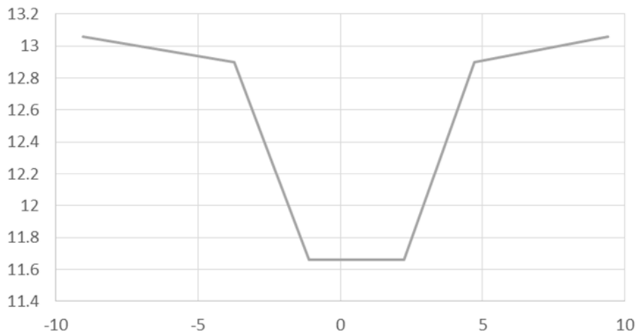
Figuur 4-4: Beekprofiel ten behoeve van beschaduwing voor de bij Bosbeekjuffer
