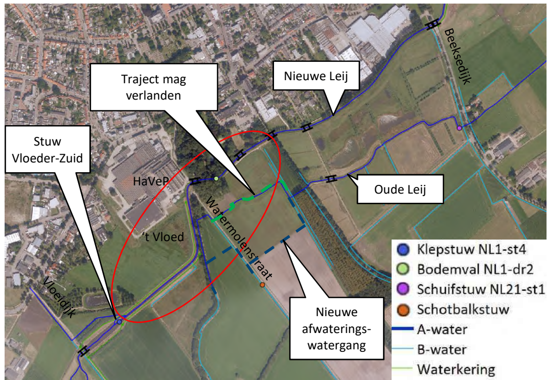
Figuur 4-5: Ligging van de afwateringswatergang is aangegeven met een blauwe stippellijn en verlanden Oude Leij met een groene stippellijn
