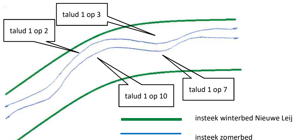
Figuur 3-5: Meandering zomerbed binnen winterbed
