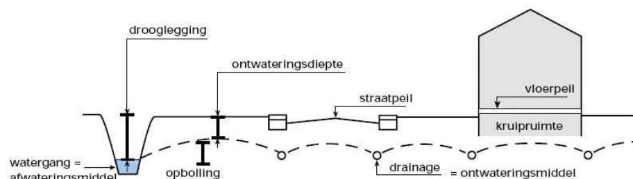
Figuur 3-4: Schematische weergave ontwateringsdiepte.
