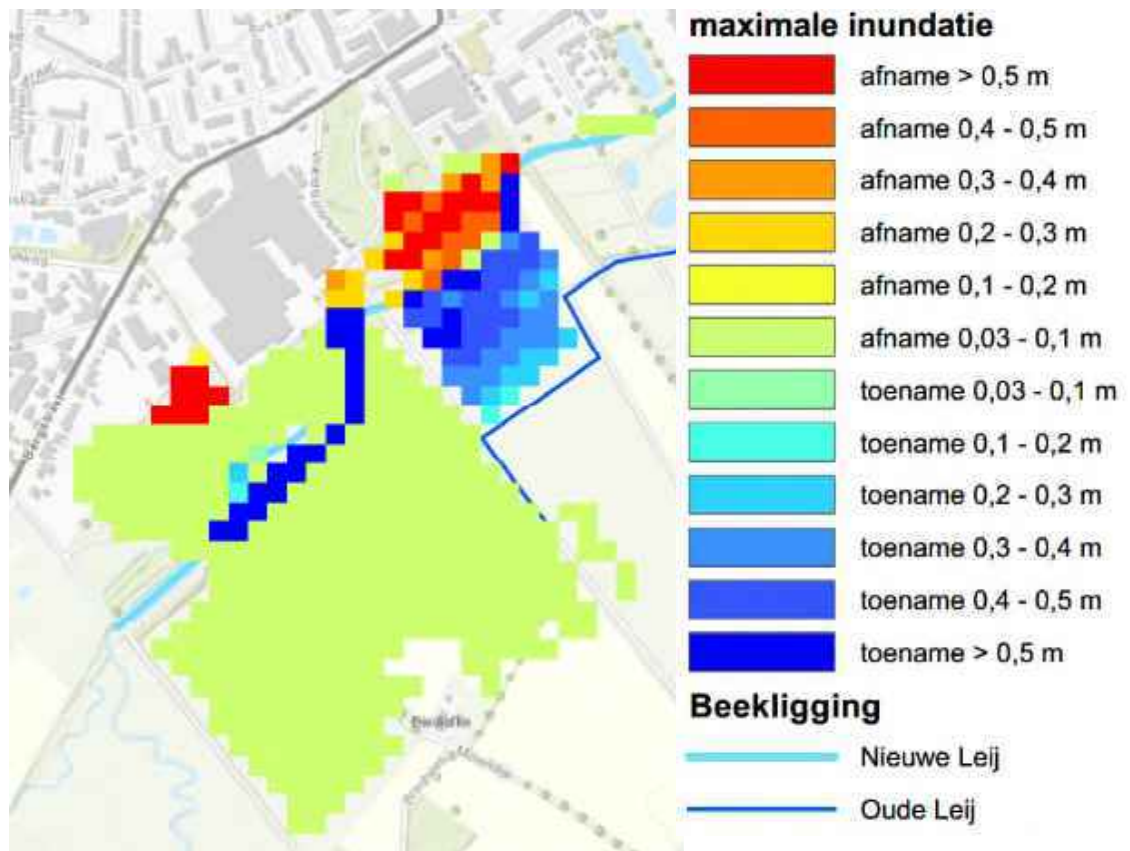
Figuur 5-5: Verschil in inundatie bij een hydrologische situatie T=100
