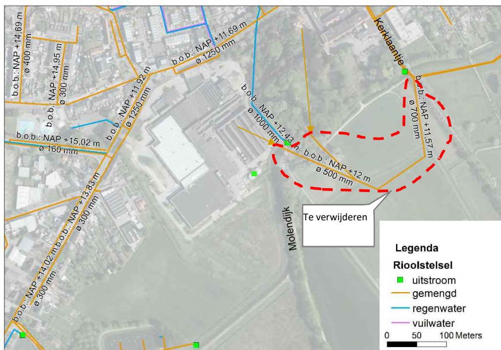
Figuur 5-7: Ligging van de riolering (bron: Gemeente Goirle)
