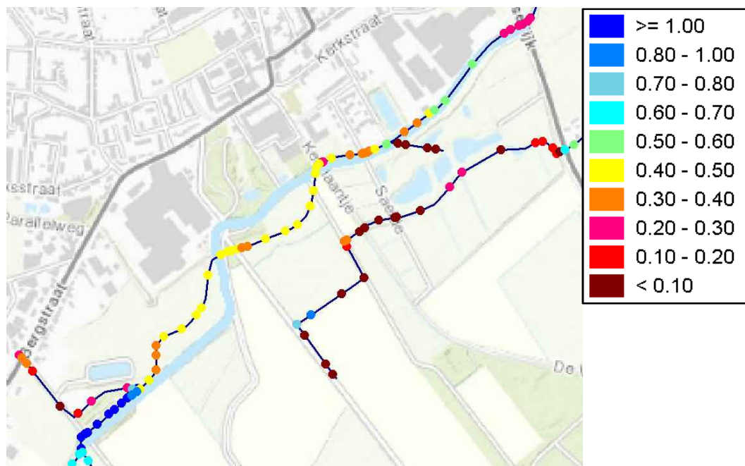
Figuur 5-2: Waterdiepte in de toekomstige situatie bij zomerafvoer
