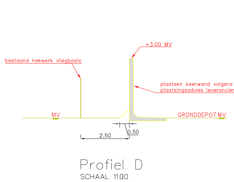
Overzicht SCHAAL 1:500
