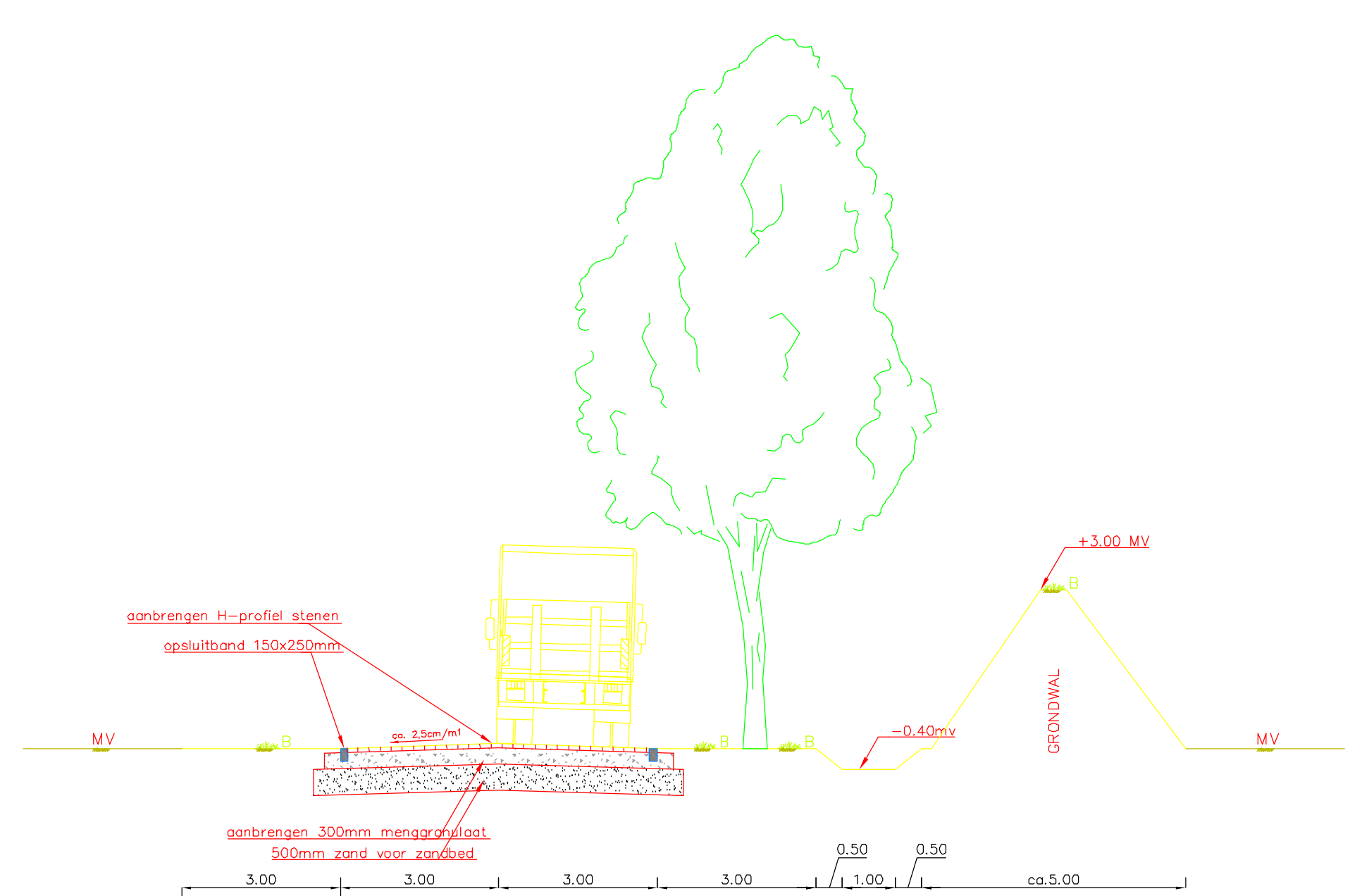
Profiel F SCHAAL 1:100
